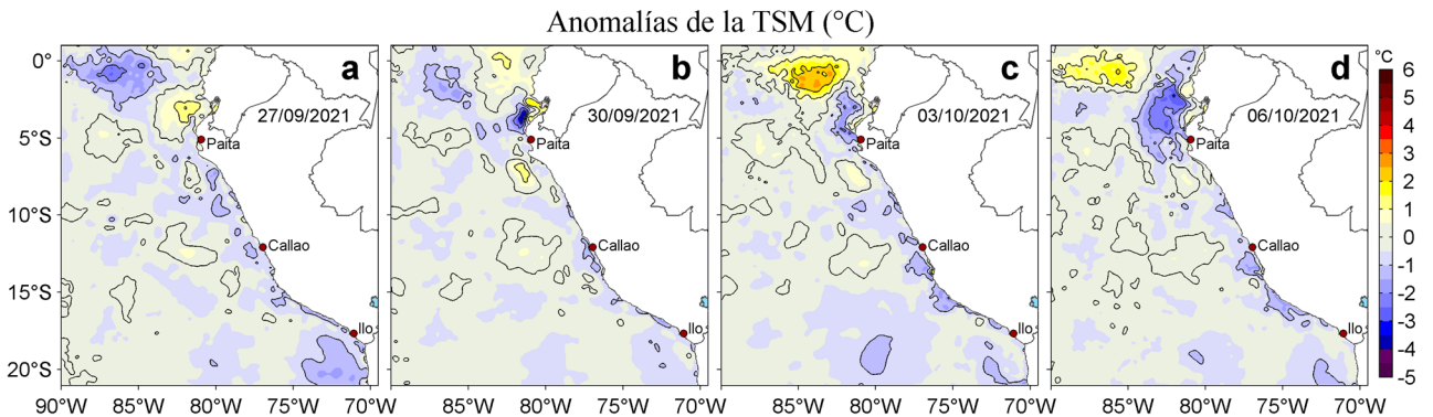
Figura 3. Anomalías de la temperatura superficial del mar (TSM, °C) para los días: a) 27 y b) 30 de setiembre, c) 03 y d) 06 de octubre de 2021. Las anomalías se calcularon respecto de la climatología para el periodo 2007-2016. Datos: OSTIA-UKMO-L4-GLOB-v2.0 (UK Met Office, 2012; Donlon et al, 2012).
