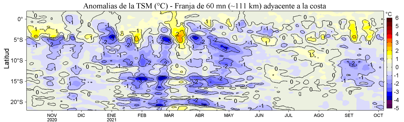
Figura 4. Variación promedio de las anomalías de la temperatura superficial del mar (TSM, °C) para una franja de 60 m.n. (~111 km) adyacente al litoral peruano para los últimos doce meses al 06 de octubre de 2021. Datos: OSTIA-UKMO-L4-GLOB-v2.0 (UK Met. Office, 2012; Donlon et al, 2012) disponible en https://podaac.jpl.nasa.gov/dataset/OSTIA-UKMO-L4-GLOB-v2.0 . Las anomalías se calcularon con respecto al periodo 2007-2016.
