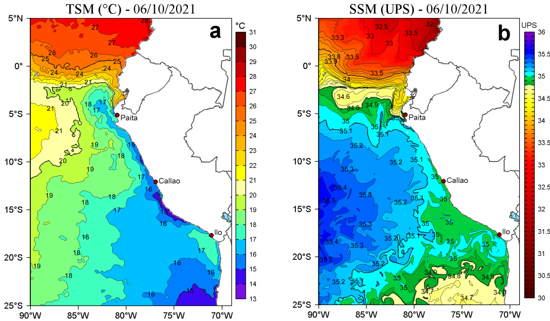
Figura 2. a) Temperatura superficial del mar (TSM, °C) y b) Salinidad superficial del mar (SSM) para el 06 de octubre de 2021. Datos: OSTIA-UKMO-L4-GLOB-v2.0 (UK Met Office, 2012; Donlon et al, 2012) disponible en https://podaac.jpl.nasa.gov/dataset/OSTIA-UKMO-L4-GLOB-v2.0 para (a) y Hybrid Coordinate Ocean Model v. GOFS 3.1 (HYCOM; Halliwell et al., 1998; 2000; Bleck, 2001) para (b).
