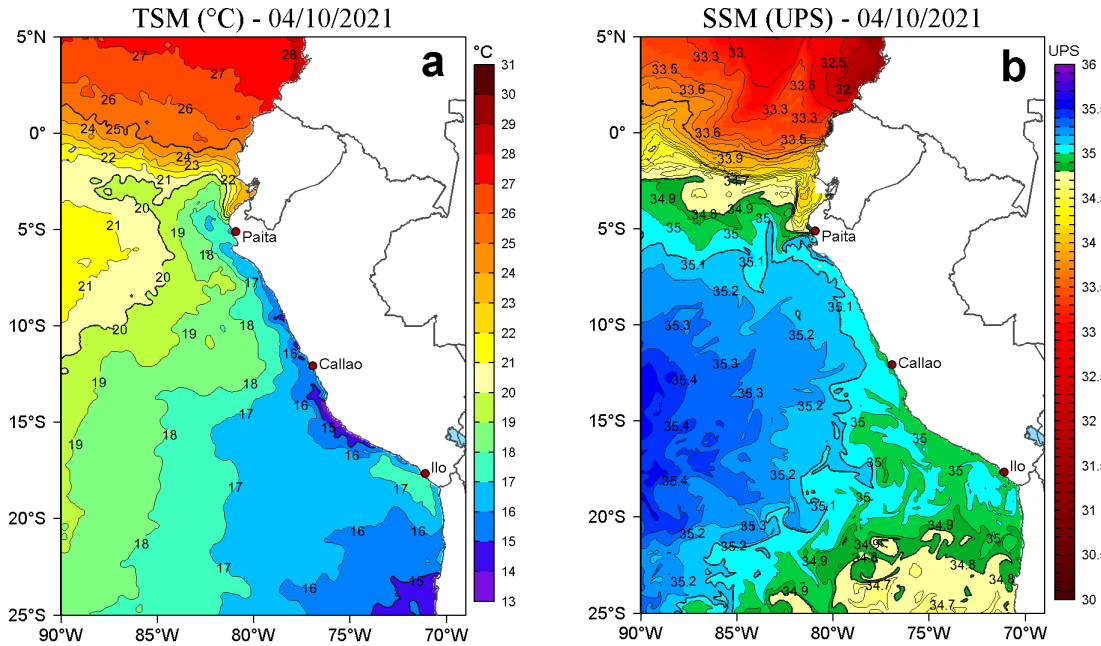
Figura 2. a) Temperatura superficial del mar (TSM, °C) y b) Salinidad superficial del mar (SSM) para el 04 de octubre de 2021. Datos: OSTIA-UKMO-L4-GLOB-v2.0 (UK Met Office, 2012; Donlon et al, 2012) disponible en https://podaac.jpl.nasa.gov/dataset/OSTIA-UKMO-L4-GLOB-v2.0 para (a) y Hybrid Coordinate Ocean Model v. GOMS 3.1 (HYCOM; Halliwell et al., 1998; 2000; Bleck, 2001) para (b).
