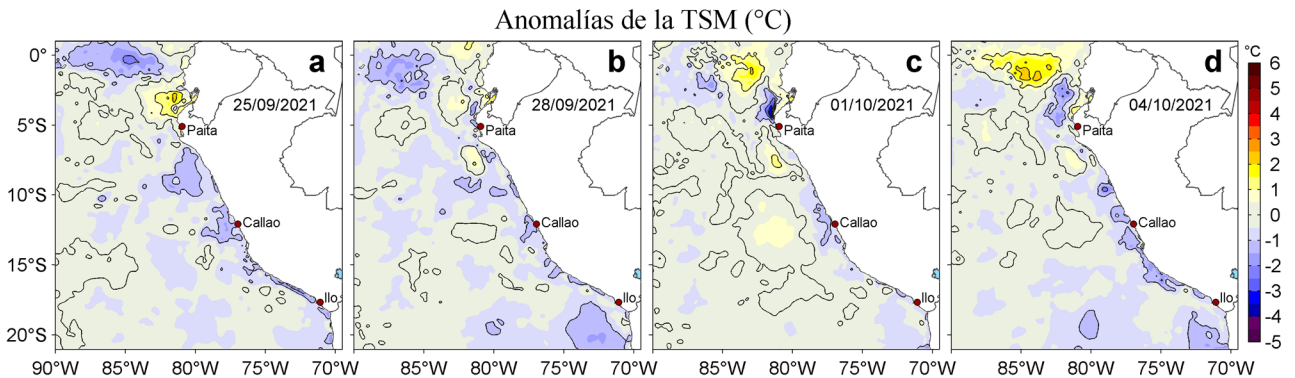
Figura 3. Anomalías de la temperatura superficial del mar (TSM, °C) para los días: a) 25 y b) 28 de setiembre, c) 01 y d) 04 de octubre de 2021. Las anomalías se calcularon respecto de la climatología para el periodo 2007-2016. Datos: OSTIA-UKMO-L4-GLOB-v2.0 (UK Met Office, 2012; Donlon et al, 2012).
