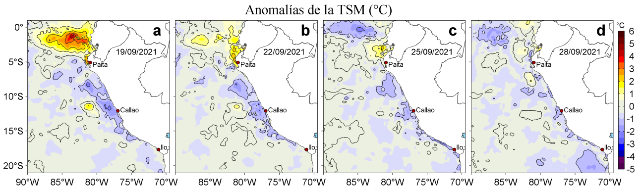
Figura 3. Anomalías de la temperatura superficial del mar (TSM, °C) para los días: a) 19, b) 22, c) 25 y d) 28 de setiembre de 2021. Las anomalías se calcularon respecto de la climatología para el periodo 2007-2016. Datos: OSTIA-UKMO-L4-GLOB-v2.0 (UK Met Office, 2012; Donlon et al, 2012).
