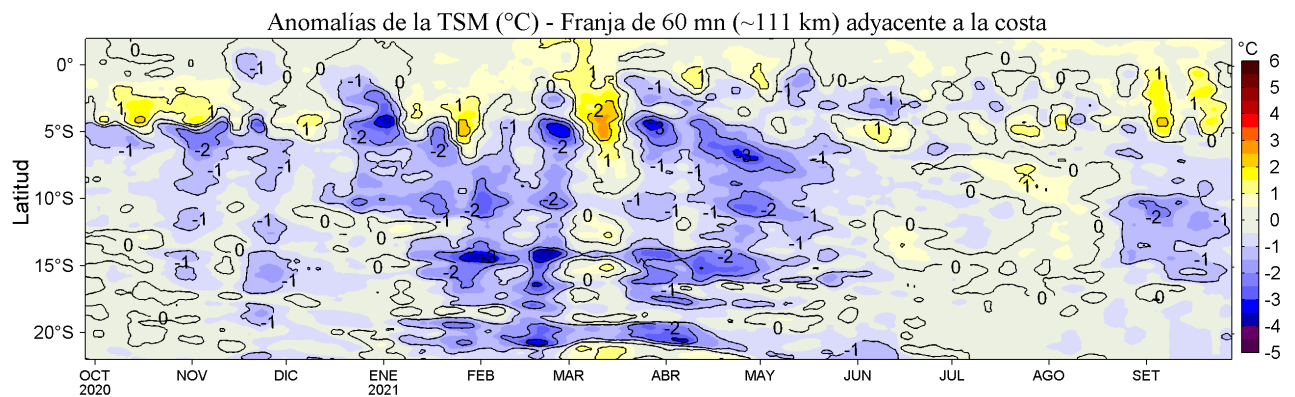
Figura 4. Variación promedio de las anomalías de la temperatura superficial del mar (TSM, °C) para una franja de 60 m.n. (~111 km) adyacente al litoral peruano para los últimos doce meses al 28 de setiembre de 2021. Datos: OSTIA-UKMO-L4-GLOB-v2.0 (UK Met. Office, 2012; Donlon et al, 2012) disponible en https://podaac.jpl.nasa.gov/dataset/OSTIA-UKMO-L4-GLOB-v2.0 . Las anomalías se calcularon con respecto al periodo 2007-2016.
