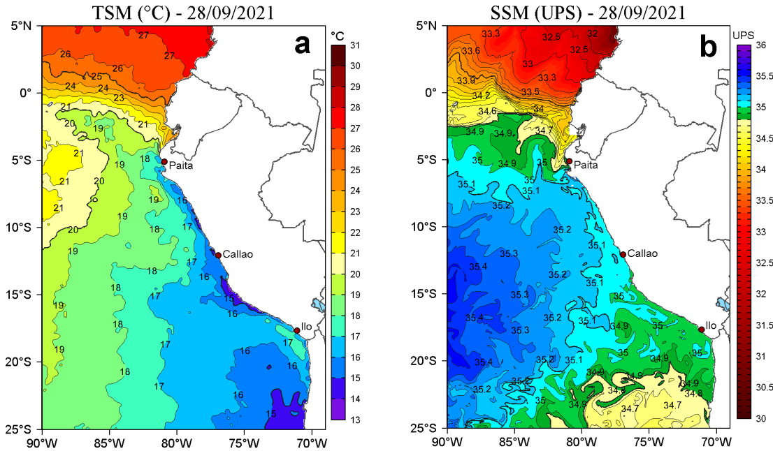
Figura 2. a) Temperatura superficial del mar (TSM, °C) y b) Salinidad superficial del mar (SSM) para el 28 de setiembre de 2021. Datos: OSTIA-UKMO-L4-GLOB-v2.0 (UK Met Office, 2012; Donlon et al, 2012) disponible en https://podaac.jpl.nasa.gov/dataset/OSTIA-UKMO-L4-GLOB-v2.0 para (a) y Hybrid Coordinate Ocean Model v. GOFS 3.1 (HYCOM; Halliwell et al., 1998; 2000; Bleck, 2001) para (b).
