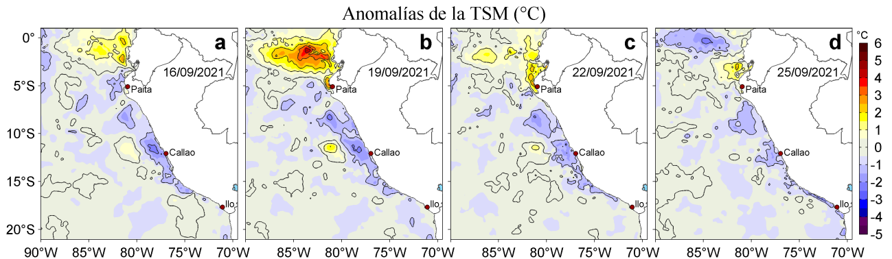
Figura 3. Anomalías de la temperatura superficial del mar (TSM, °C) para los días: a) 16, b) 19, c) 22 y d) 25 de setiembre de 2021. Las anomalías se calcularon respecto de la climatología para el periodo 2007-2016. Datos: OSTIA-UKMO-L4-GLOB-v2.0 (UK Met Office, 2012; Donlon et al, 2012).
