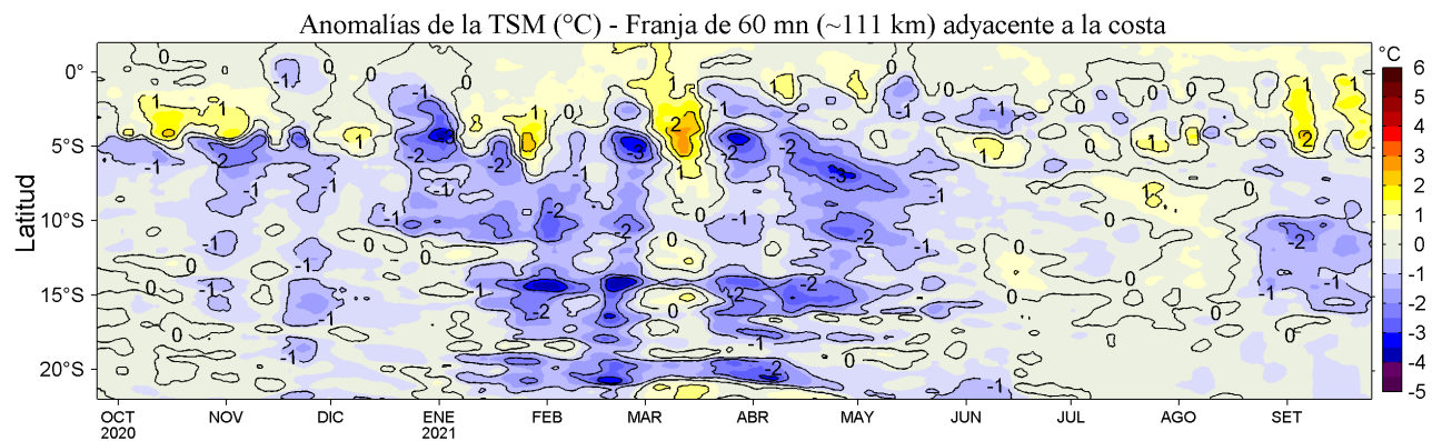
Figura 4. Variación promedio de las anomalías de la temperatura superficial del mar (TSM, °C) para una franja de 60 m.n. (~111 km) adyacente al litoral peruano para los últimos doce meses al 25 de setiembre de 2021. Datos: OSTIA-UKMO-L4-GLOB-v2.0 (UK Met. Office, 2012; Donlon et al, 2012) disponible en https://podaac.jpl.nasa.gov/dataset/OSTIA-UKMO-L4-GLOB-v2.0 . Las anomalías se calcularon con respecto al periodo 2007-2016.
