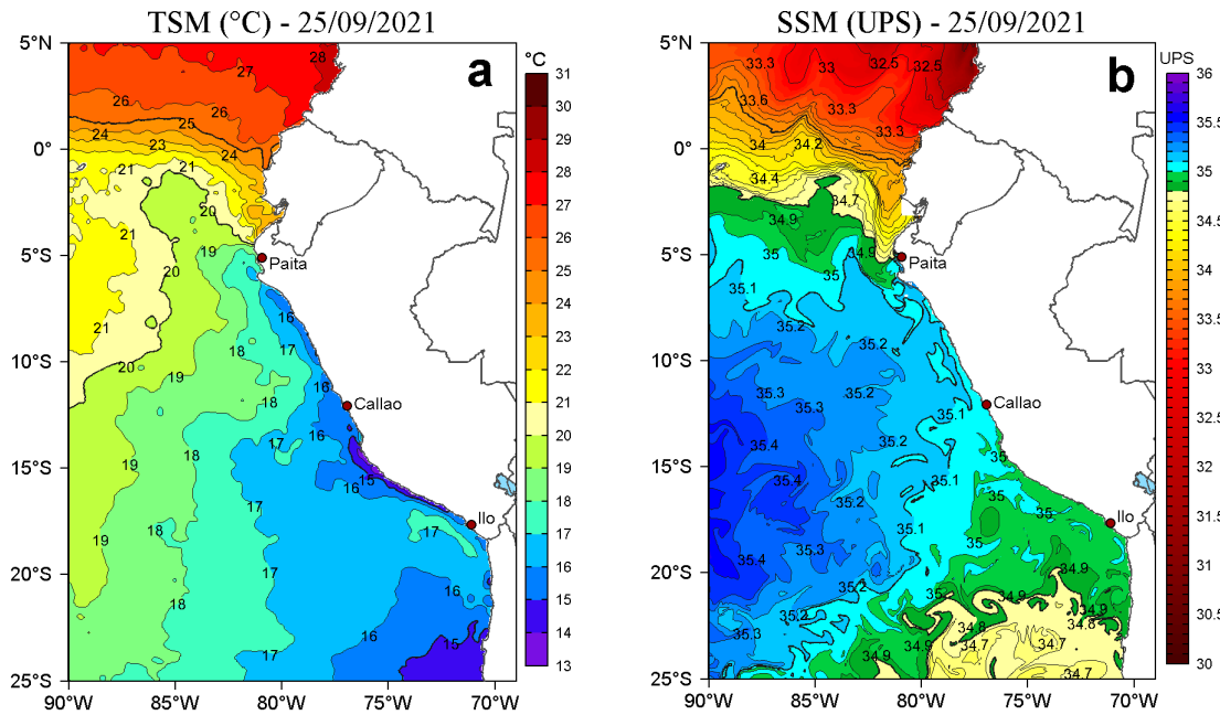
Figura 2. a) Temperatura superficial del mar (TSM, °C) y b) Salinidad superficial del mar (SSM) para el 25 de setiembre de 2021. Datos: OSTIA-UKMO-L4-GLOB-v2.0 (UK Met Office, 2012; Donlon et al, 2012) disponible en https://podaac.jpl.nasa.gov/dataset/OSTIA-UKMO-L4-GLOB-v2.0 para (a) y Hybrid Coordinate Ocean Model v. GOFS 3.1 (HYCOM; Halliwell et al., 1998; 2000; Bleck, 2001) para (b).
