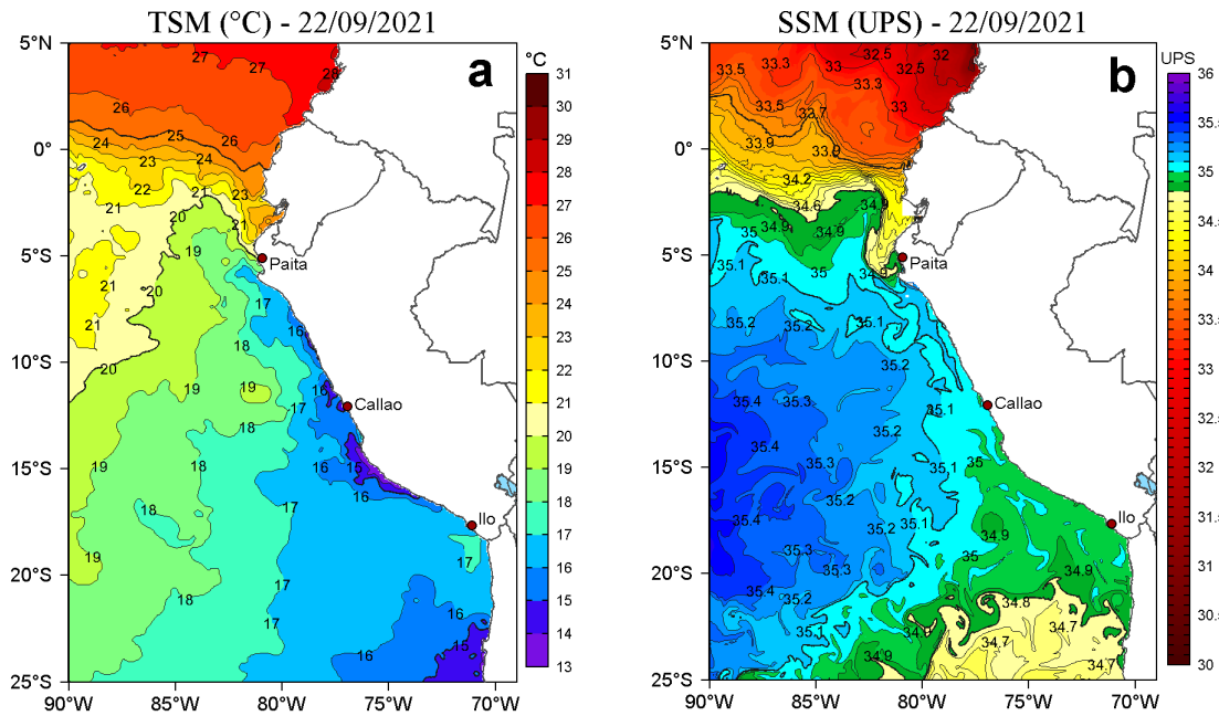
Figura 2. a) Temperatura superficial del mar (TSM, °C) y b) Salinidad superficial del mar (SSM) para el 22 de setiembre de 2021. Datos: OSTIA-UKMO-L4-GLOB-v2.0 (UK Met Office, 2012; Donlon et al, 2012) disponible en https://podaac.jpl.nasa.gov/dataset/OSTIA-UKMO-L4-GLOB-v2.0 para (a) y Hybrid Coordinate Ocean Model v. GOFS 3.1 (HYCOM; Halliwell et al., 1998; 2000; Bleck, 2001) para (b).
