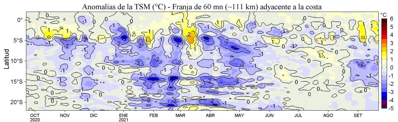
Figura 4. Variación promedio de las anomalías de la temperatura superficial del mar (TSM, °C) para una franja de 60 m.n. (~111 km) adyacente al litoral peruano para los últimos doce meses al 22 de setiembre de 2021. Datos: OSTIA-UKMO-L4-GLOB-v2.0 (UK Met. Office, 2012; Donlon et al, 2012) disponible en https://podaac.jpl.nasa.gov/dataset/OSTIA-UKMO-L4-GLOB-v2.0 . Las anomalías se calcularon con respecto al periodo 2007-2016.
