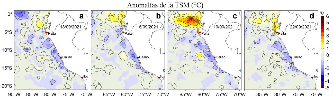
Figura 3. Anomalías de la temperatura superficial del mar (TSM, °C) para los días: a) 13, b) 16, c) 19 y d) 22 de setiembre de 2021. Las anomalías se calcularon respecto de la climatología para el periodo 2007-2016. Datos: OSTIA-UKMO-L4-GLOB-v2.0 (UK Met Office, 2012; Donlon et al, 2012).
