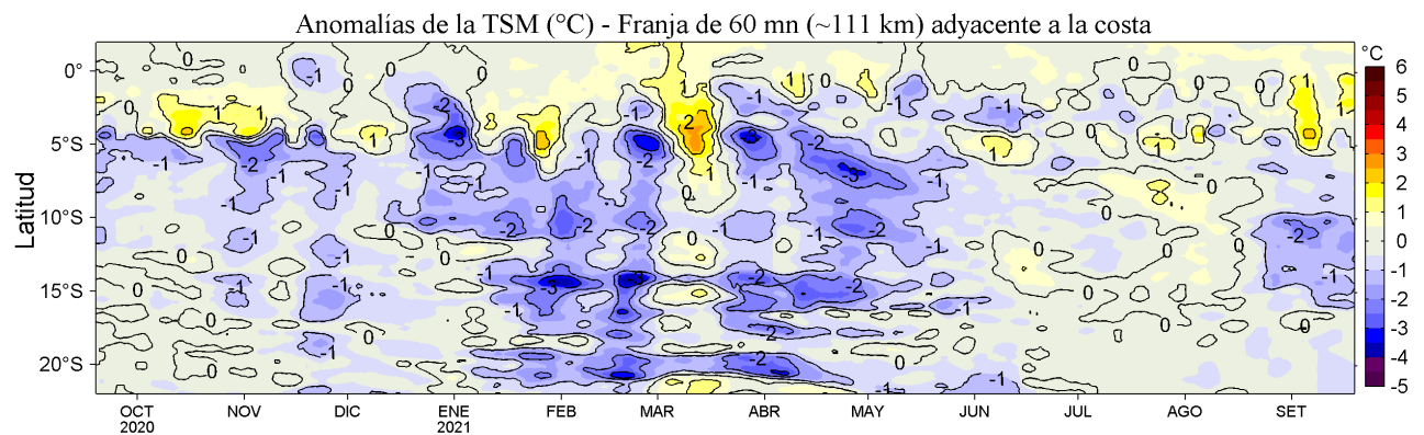
Figura 4. Variación promedio de las anomalías de la temperatura superficial del mar (TSM, °C) para una franja de 60 m.n. (~111 km) adyacente al litoral peruano para los últimos doce meses al 19 de setiembre de 2021. Datos: OSTIA-UKMO-L4-GLOB-v2.0 (UK Met. Office, 2012; Donlon et al, 2012) disponible en https://podaac.jpl.nasa.gov/dataset/OSTIA-UKMO-L4-GLOB-v2.0 . Las anomalías se calcularon con respecto al periodo 2007-2016.
