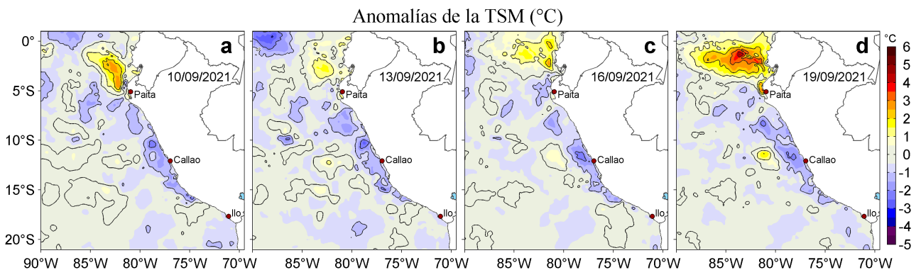
Figura 3. Anomalías de la temperatura superficial del mar (TSM, °C) para los días: a) 10, b) 13, c) 16 y d) 19 de setiembre de 2021. Las anomalías se calcularon respecto de la climatología para el periodo 2007-2016. Datos: OSTIA-UKMO-L4-GLOB-v2.0 (UK Met Office, 2012; Donlon et al, 2012).
