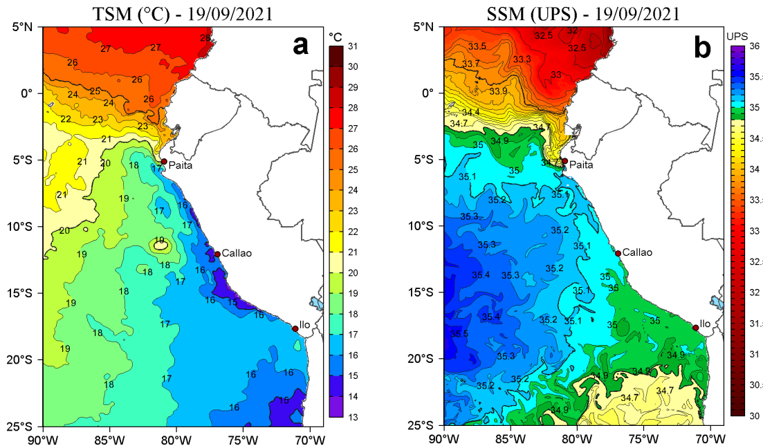
Figura 2. a) Temperatura superficial del mar (TSM, °C) y b) Salinidad superficial del mar (SSM) para el 19 de setiembre de 2021. Datos: OSTIA-UKMO-L4-GLOB-v2.0 (UK Met Office, 2012; Donlon et al, 2012) disponible en https://podaac.jpl.nasa.gov/dataset/OSTIA-UKMO-L4-GLOB-v2.0 para (a) y Hybrid Coordinate Ocean Model v. GOFS 3.1 (HYCOM; Halliwell et al., 1998; 2000; Bleck, 2001) para (b).
