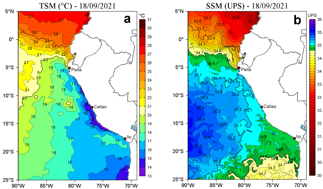
Figura 2. a) Temperatura superficial del mar (TSM, °C) y b) Salinidad superficial del mar (SSM) para el 18 de setiembre de 2021. Datos: OSTIA-UKMO-L4-GLOB-v2.0 (UK Met Office, 2012; Donlon et al, 2012) disponible en https://podaac.jpl.nasa.gov/dataset/OSTIA-UKMO-L4-GLOB-v2.0 para (a) y Hybrid Coordinate Ocean Model v. GOFS 3.1 (HYCOM; Halliwell et al., 1998; 2000; Bleck, 2001) para (b).
