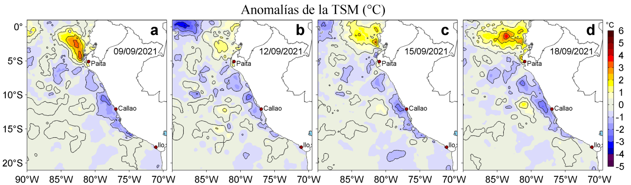
Figura 3. Anomalías de la temperatura superficial del mar (TSM, °C) para los días: a) 09, b) 12, c) 15 y d) 18 de setiembre de 2021. Las anomalías se calcularon respecto de la climatología para el periodo 2007-2016. Datos: OSTIA-UKMO-L4-GLOB-v2.0 (UK Met Office, 2012; Donlon et al, 2012).
