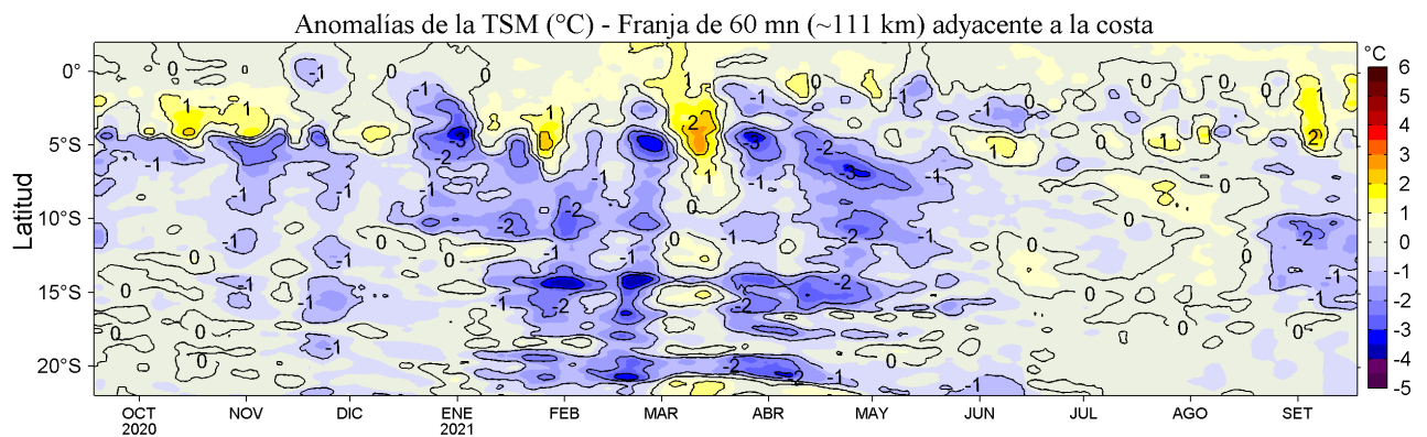
Figura 4. Variación promedio de las anomalías de la temperatura superficial del mar (TSM, °C) para una franja de 60 m.n. (~111 km) adyacente al litoral peruano para los últimos doce meses al 18 de setiembre de 2021. Datos: OSTIA-UKMO-L4-GLOB-v2.0 (UK Met. Office, 2012; Donlon et al, 2012) disponible en https://podaac.jpl.nasa.gov/dataset/OSTIA-UKMO-L4-GLOB-v2.0 . Las anomalías se calcularon con respecto al periodo 2007-2016.
