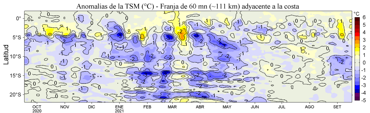
Figura 4. Variación promedio de las anomalías de la temperatura superficial del mar (TSM, °C) para una franja de 60 m.n. (~111 km) adyacente al litoral peruano para los últimos doce meses al 17 de setiembre de 2021. Datos: OSTIA-UKMO-L4-GLOB-v2.0 (UK Met. Office, 2012; Donlon et al, 2012) disponible en https://podaac.jpl.nasa.gov/dataset/OSTIA-UKMO-L4-GLOB-v2.0 . Las anomalías se calcularon con respecto al periodo 2007-2016.
