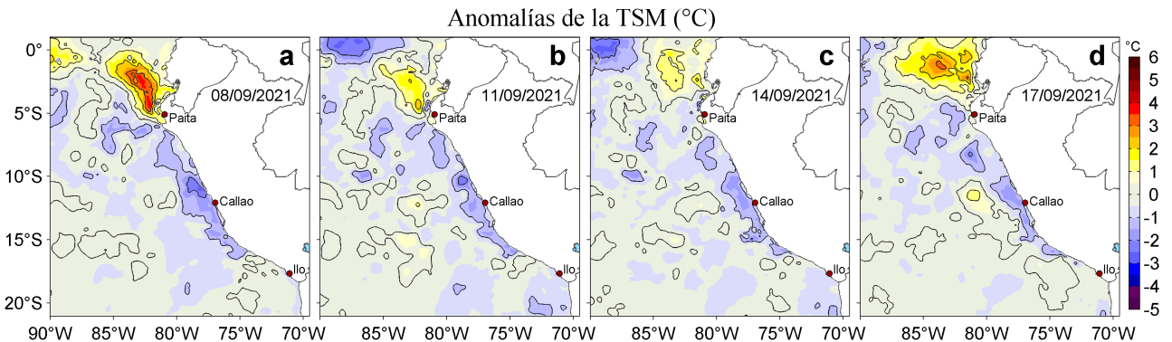
Figura 3. Anomalías de la temperatura superficial del mar (TSM, °C) para los días: a) 08, b) 11, c) 14 y d) 17 de setiembre de 2021. Las anomalías se calcularon respecto de la climatología para el periodo 2007-2016. Datos: OSTIA-UKMO-L4-GLOB-v2.0 (UK Met Office, 2012; Donlon et al, 2012).
