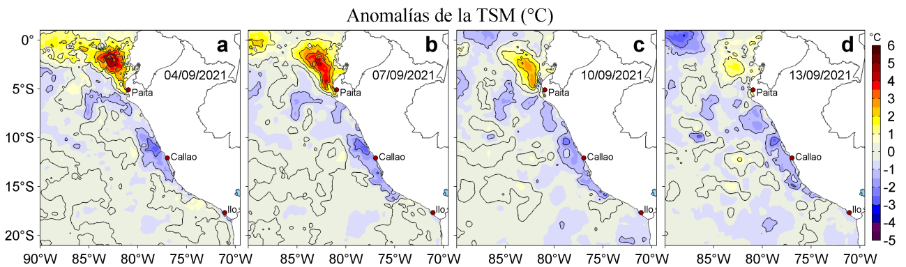
Figura 3. Anomalías de la temperatura superficial del mar (TSM, °C) para los días: a) 04, b) 07, c) 10 y d) 13 de setiembre de 2021. Las anomalías se calcularon respecto de la climatología para el periodo 2007-2016. Datos: OSTIA-UKMO-L4-GLOB-v2.0 (UK Met Office, 2012; Donlon et al, 2012).
