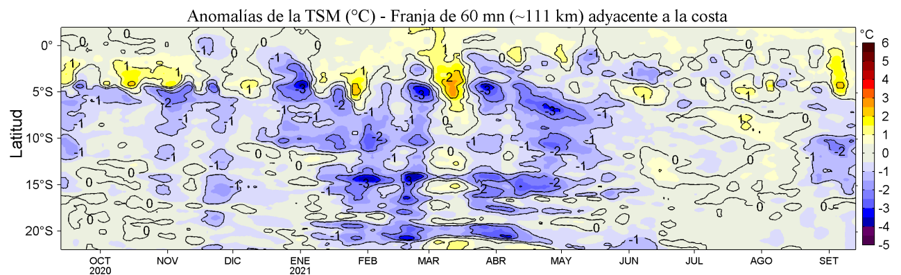
Figura 4. Variación promedio de las anomalías de la temperatura superficial del mar (TSM, °C) para una franja de 60 m.n. (~111 km) adyacente al litoral peruano para los últimos doce meses al 13 de setiembre de 2021. Datos: OSTIA-UKMO-L4-GLOB-v2.0 (UK Met. Office, 2012; Donlon et al, 2012) disponible en https://podaac.jpl.nasa.gov/dataset/OSTIA-UKMO-L4-GLOB-v2.0 . Las anomalías se calcularon con respecto al periodo 2007-2016.
