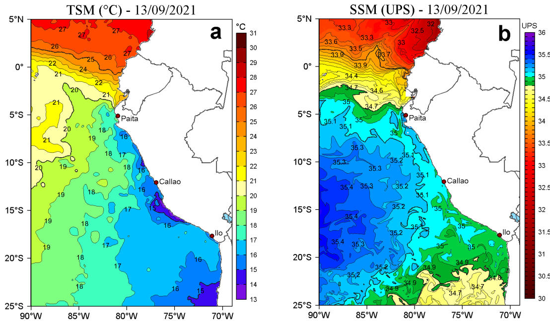
Figura 2. a) Temperatura superficial del mar (TSM, °C) y b) Salinidad superficial del mar (SSM) para el 13 de setiembre de 2021. Datos: OSTIA-UKMO-L4-GLOB-v2.0 (UK Met Office, 2012; Donlon et al, 2012) disponible en https://podaac.jpl.nasa.gov/dataset/OSTIA-UKMO-L4-GLOB-v2.0 para (a) y Hybrid Coordinate Ocean Model v. GOF5 3.1 (HYCOM; Halliwell et al., 1998; 2000; Bleck, 2001) para (b).
