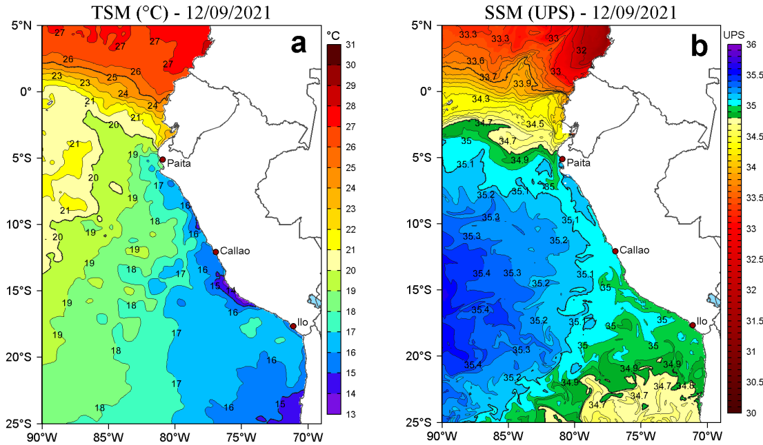
Figura 2. a) Temperatura superficial del mar (TSM, °C) y b) Salinidad superficial del mar (SSM) para el 12 de setiembre de 2021. Datos: OSTIA-UKMO-L4-GLOB-v2.0 (UK Met Office, 2012; Donlon et al, 2012) disponible en https://podaac.jpl.nasa.gov/dataset/OSTIA-UKMO-L4-GLOB-v2.0 para (a) y Hybrid Coordinate Ocean Model v. GOFS 3.1 (HYCOM; Halliwell et al., 1998; 2000; Bleck, 2001) para (b).
