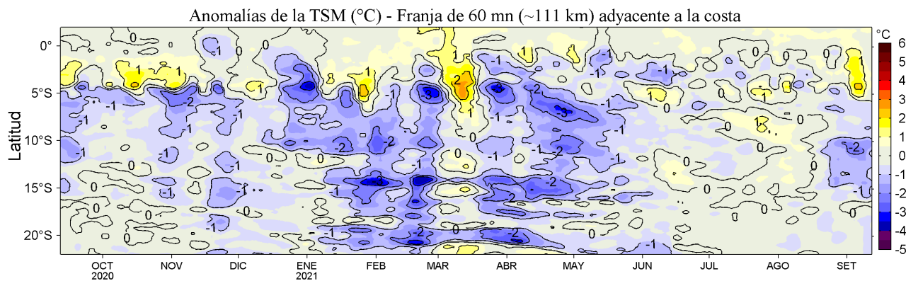
Figura 4. Variación promedio de las anomalías de la temperatura superficial del mar (TSM, °C) para una franja de 60 m.n. (~111 km) adyacente al litoral peruano para los últimos doce meses al 12 de setiembre de 2021. Datos: OSTIA-UKMO-L4-GLOB-v2.0 (UK Met. Office, 2012; Donlon et al, 2012) disponible en https://podaac.jpl.nasa.gov/dataset/OSTIA-UKMO-L4-GLOB-v2.0 . Las anomalías se calcularon con respecto al periodo 2007-2016.
