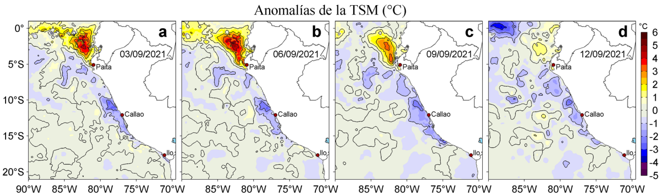
Figura 3. Anomalías de la temperatura superficial del mar (TSM, °C) para los días: a) 03, b) 06, c) 09 y d) 12 de setiembre de 2021. Las anomalías se calcularon respecto de la climatología para el periodo 2007-2016. Datos: OSTIA-UKMO-L4-GLOB-v2.0 (UK Met Office, 2012; Donlon et al, 2012).
