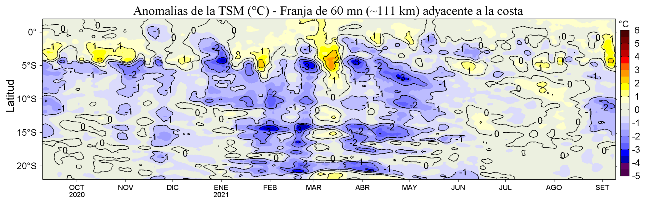
Figura 4. Variación promedio de las anomalías de la temperatura superficial del mar (TSM, °C) para una franja de 60 m.n. (~111 km) adyacente al litoral peruano para los últimos doce meses al 09 de setiembre de 2021. Datos: OSTIA-UKMO-L4-GLOB-v2.0 (UK Met. Office, 2012; Donlon et al, 2012) disponible en https://podaac.jpl.nasa.gov/dataset/OSTIA-UKMO-L4-GLOB-v2.0 . Las anomalías se calcularon con respecto al periodo 2007-2016.
