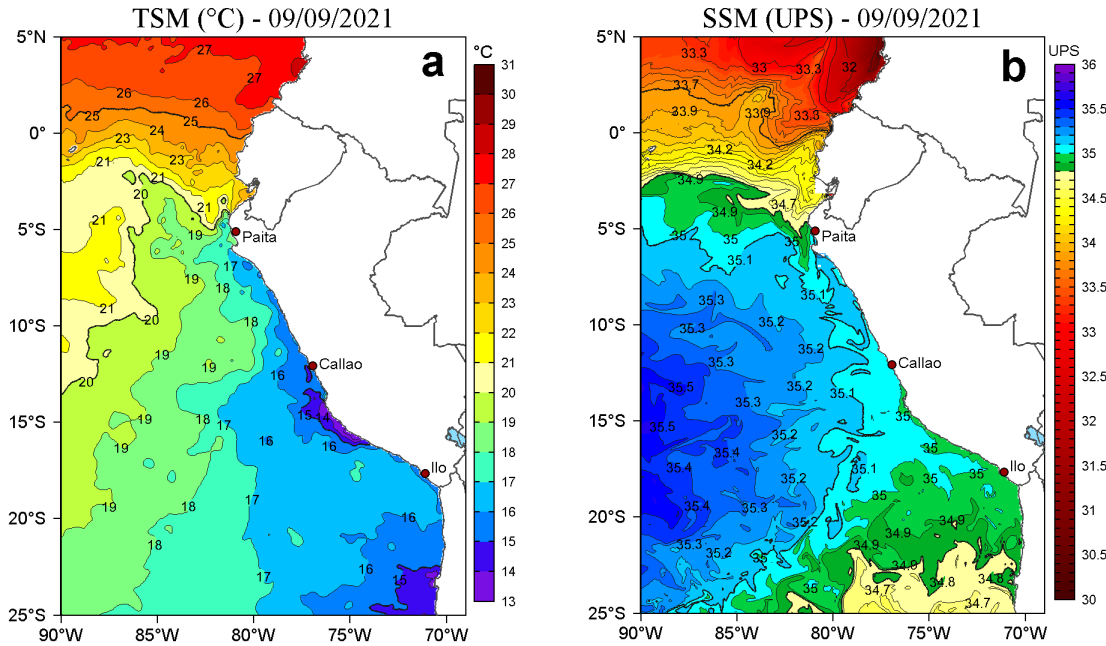
Figura 2. a) Temperatura superficial del mar (TSM, °C) y b) Salinidad superficial del mar (SSM) para el 09 de setiembre de 2021. Datos: OSTIA-UKMO-L4-GLOB-v2.0 (UK Met Office, 2012; Donlon et al, 2012) disponible en https://podaac.jpl.nasa.gov/dataset/OSTIA-UKMO-L4-GLOB-v2.0 para (a) y Hybrid Coordinate Ocean Model v. GOFS 3.1 (HYCOM; Halliwell et al., 1998; 2000; Bleck, 2001) para (b).
