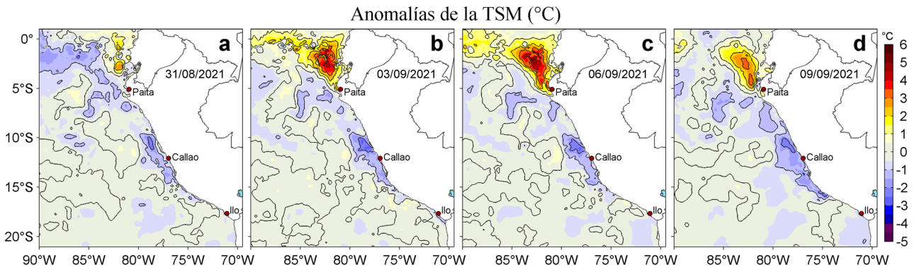
Figura 3. Anomalías de la temperatura superficial del mar (TSM, °C) para los días: a) 31 de agosto, b) 03, c) 06 y d) 09 de setiembre de 2021. Las anomalías se calcularon respecto de la climatología para el periodo 2007-2016. Datos: OSTIA-UKMO-L4-GLOB-v2.0 (UK Met Office, 2012; Donlon et al, 2012).
