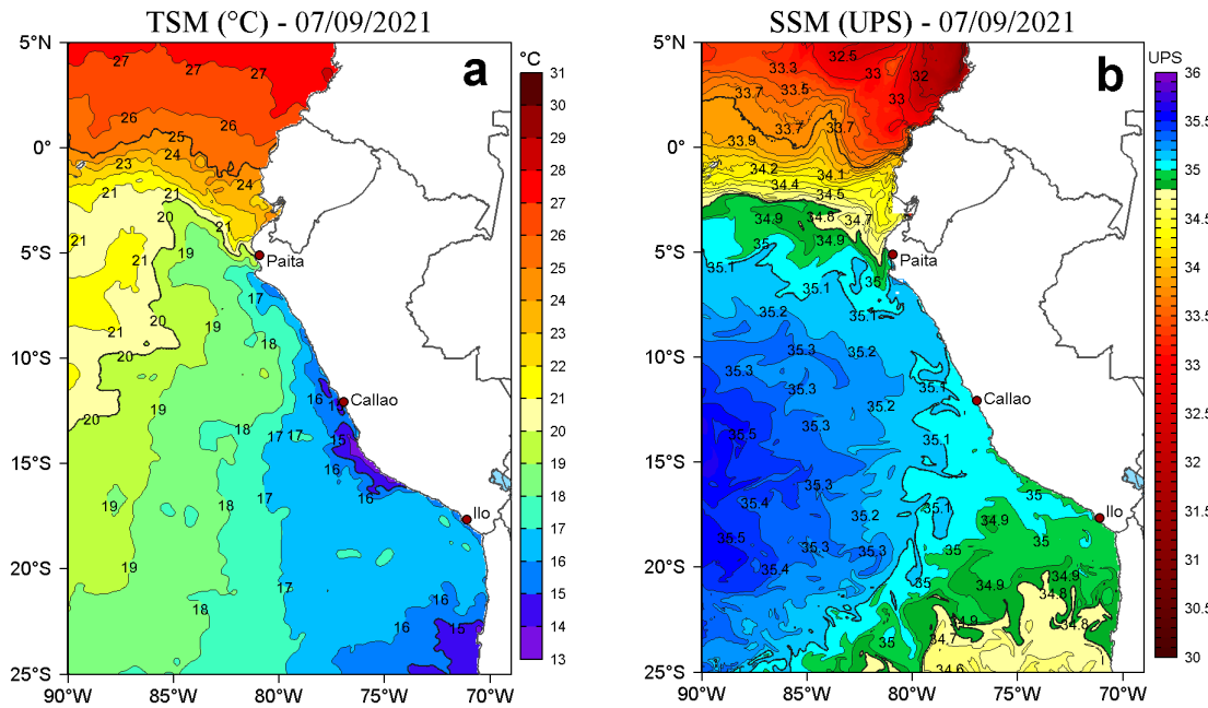
Figura 2. a) Temperatura superficial del mar (TSM, °C) y b) Salinidad superficial del mar (SSM) para el 07 de setiembre de 2021. Datos: OSTIA-UKMO-L4-GLOB-v2.0 (UK Met Office, 2012; Donlon et al, 2012) disponible en https://podaac.jpl.nasa.gov/dataset/OSTIA-UKMO-L4-GLOB-v2.0 para (a) y Hybrid Coordinate Ocean Model v. GOFS 3.1 (HYCOM; Halliwell et al., 1998; 2000; Bleck, 2001) para (b).
