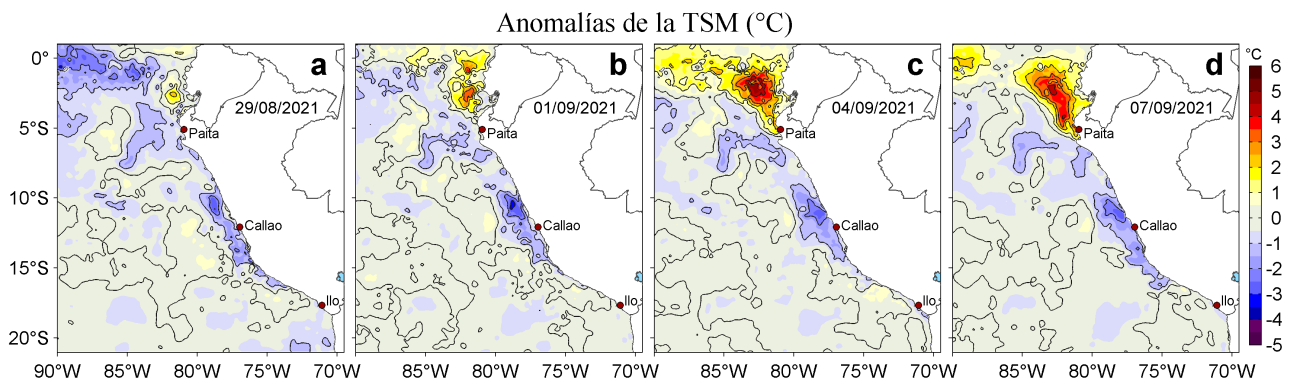
Figura 3. Anomalías de la temperatura superficial del mar (TSM, °C) para los días: a) 29 de agosto, b) 01, c) 04 y d) 07 de setiembre de 2021. Las anomalías se calcularon respecto de la climatología para el periodo 2007-2016. Datos: OSTIA-UKMO-L4-GLOB-v2.0 (UK Met Office, 2012; Donlon et al, 2012).
