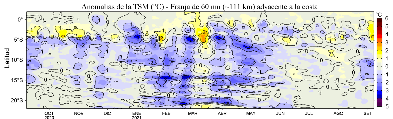
Figura 4. Variación promedio de las anomalías de la temperatura superficial del mar (TSM, °C) para una franja de 60 m.n. (~111 km) adyacente al litoral peruano para los últimos doce meses al 07 de setiembre de 2021. Datos: OSTIA-UKMO-L4-GLOB-v2.0 (UK Met. Office, 2012; Donlon et al, 2012) disponible en https://podaac.jpl.nasa.gov/dataset/OSTIA-UKMO-L4-GLOB-v2.0 . Las anomalías se calcularon con respecto al periodo 2007-2016.
