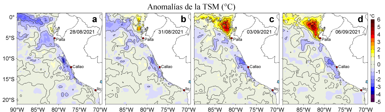
Figura 3. Anomalías de la temperatura superficial del mar (TSM, °C) para los días: a) 28 y b) 31 de agosto, c) 03 y d) 06 de setiembre de 2021. Las anomalías se calcularon respecto de la climatología para el periodo 2007-2016. Datos: OSTIA-UKMO-L4-GLOB-v2.0 (UK Met Office, 2012; Donlon et al, 2012).
