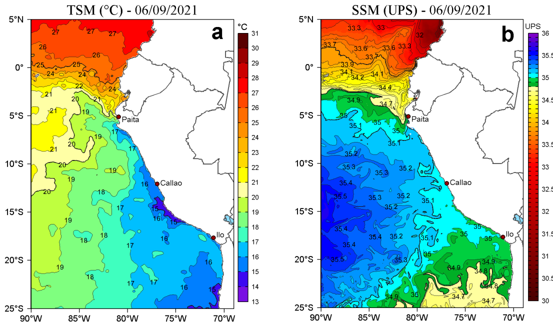
Figura 2. a) Temperatura superficial del mar (TSM, °C) y b) Salinidad superficial del mar (SSM) para el 06 de setiembre de 2021. Datos: OSTIA-UKMO-L4-GLOB-v2.0 (UK Met Office, 2012; Donlon et al, 2012) disponible en https://podaac.jpl.nasa.gov/dataset/OSTIA-UKMO-L4-GLOB-v2.0 para (a) y Hybrid Coordinate Ocean Model v. GOFS 3.1 (HYCOM; Halliwell et al., 1998; 2000; Bleck, 2001) para (b).
