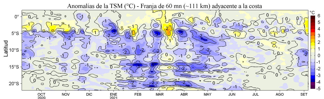
Figura 4. Variación promedio de las anomalías de la temperatura superficial del mar (TSM, °C) para una franja de 60 m.n. (~111 km) adyacente al litoral peruano para los últimos doce meses al 06 de setiembre de 2021. Datos: OSTIA-UKMO-L4-GLOB-v2.0 (UK Met. Office, 2012; Donlon et al, 2012) disponible en https://podaac.jpl.nasa.gov/dataset/OSTIA-UKMO-L4-GLOB-v2.0 . Las anomalías se calcularon con respecto al periodo 2007-2016.
