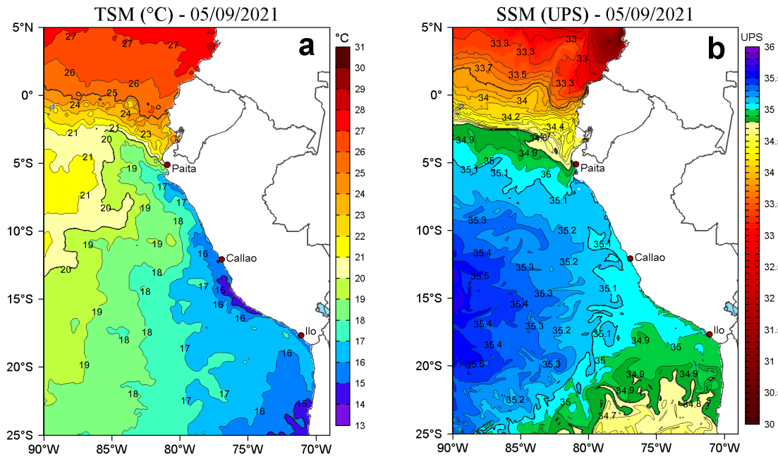
Figura 2. a) Temperatura superficial del mar (TSM, °C) y b) Salinidad superficial del mar (SSM) para el 05 de setiembre de 2021. Datos: OSTIA-UKMO-L4-GLOB-v2.0 (UK Met Office, 2012; Donlon et al, 2012) disponible en https://podaac.jpl.nasa.gov/dataset/OSTIA-UKMO-L4-GLOB-v2.0 para (a) y Hybrid Coordinate Ocean Model v. GOFS 3.1 (HYCOM; Halliwell et al., 1998; 2000; Bleck, 2001) para (b).
