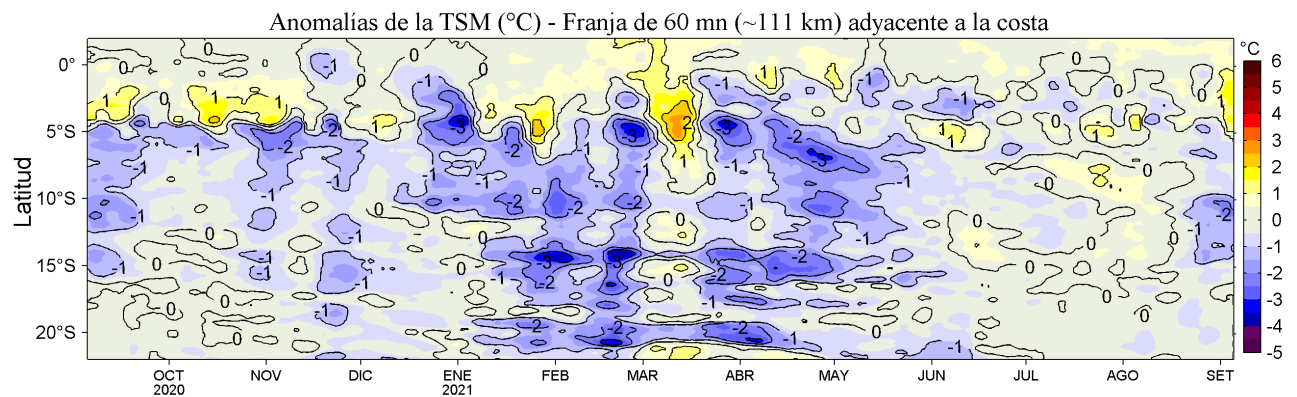
Figura 4. Variación promedio de las anomalías de la temperatura superficial del mar (TSM, °C) para una franja de 60 m.n. (~111 km) adyacente al litoral peruano para los últimos doce meses al 05 de setiembre de 2021. Datos: OSTIA-UKMO-L4-GLOB-v2.0 (UK Met. Office, 2012; Donlon et al, 2012) disponible en https://podaac.jpl.nasa.gov/dataset/OSTIA-UKMO-L4-GLOB-v2.0 . Las anomalías se calcularon con respecto al periodo 2007-2016.
