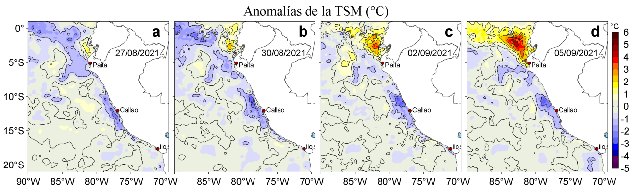
Figura 3. Anomalías de la temperatura superficial del mar (TSM, °C) para los días: a) 27 y b) 30 de agosto, c) 02 y d) 05 de setiembre de 2021. Las anomalías se calcularon respecto de la climatología para el periodo 2007-2016. Datos: OSTIA-UKMO-L4-GLOB-v2.0 (UK Met Office, 2012; Donlon et al, 2012).
