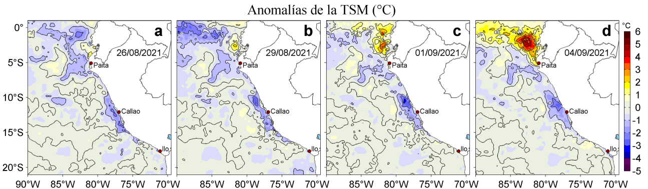
Figura 3. Anomalías de la temperatura superficial del mar (TSM, °C) para los días: a) 26 y b) 29 de agosto, c) 01 y d) 04 de setiembre de 2021. Las anomalías se calcularon respecto de la climatología para el periodo 2007-2016. Datos: OSTIA-UKMO-L4-GLOB-v2.0 (UK Met Office, 2012; Donlon et al, 2012).
