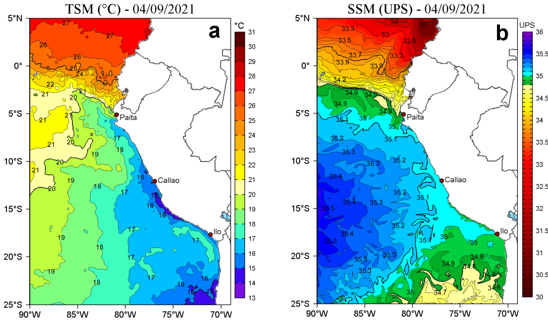
Figura 2. a) Temperatura superficial del mar (TSM, °C) y b) Salinidad superficial del mar (SSM) para el 04 de setiembre de 2021. Datos: OSTIA-UKMO-L4-GLOB-v2.0 (UK Met Office, 2012; Donlon et al, 2012) disponible en https://podaac.jpl.nasa.gov/dataset/OSTIA-UKMO-L4-GLOB-v2.0 para (a) y Hybrid Coordinate Ocean Model v. GOFS 3.1 (HYCOM; Halliwell et al., 1998; 2000; Bleck, 2001) para (b).
