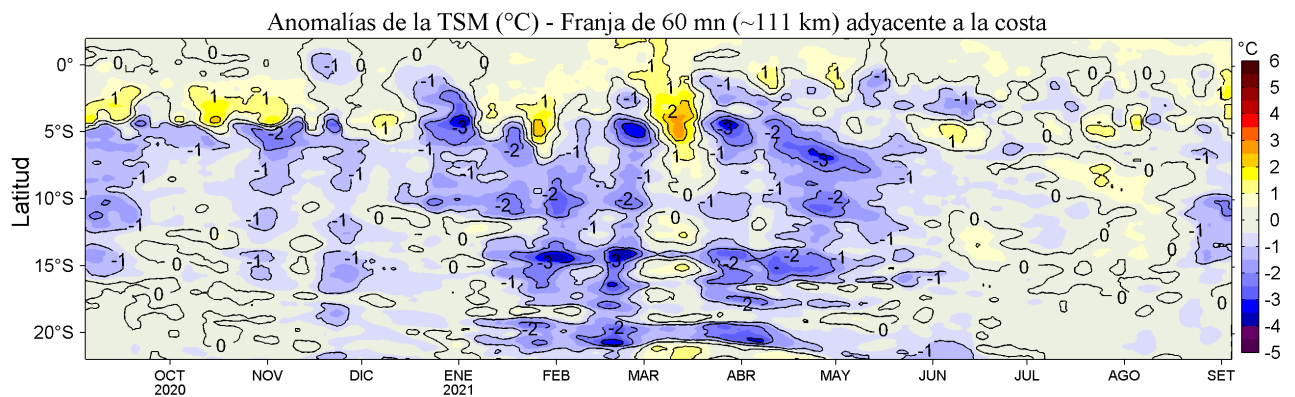
Figura 4. Variación promedio de las anomalías de la temperatura superficial del mar (TSM, °C) para una franja de 60 m.n. (~111 km) adyacente al litoral peruano para los últimos doce meses al 04 de setiembre de 2021. Datos: OSTIA-UKMO-L4-GLOB-v2.0 (UK Met. Office, 2012; Donlon et al, 2012) disponible en https://podaac.jpl.nasa.gov/dataset/OSTIA-UKMO-L4-GLOB-v2.0 . Las anomalías se calcularon con respecto al periodo 2007-2016.
