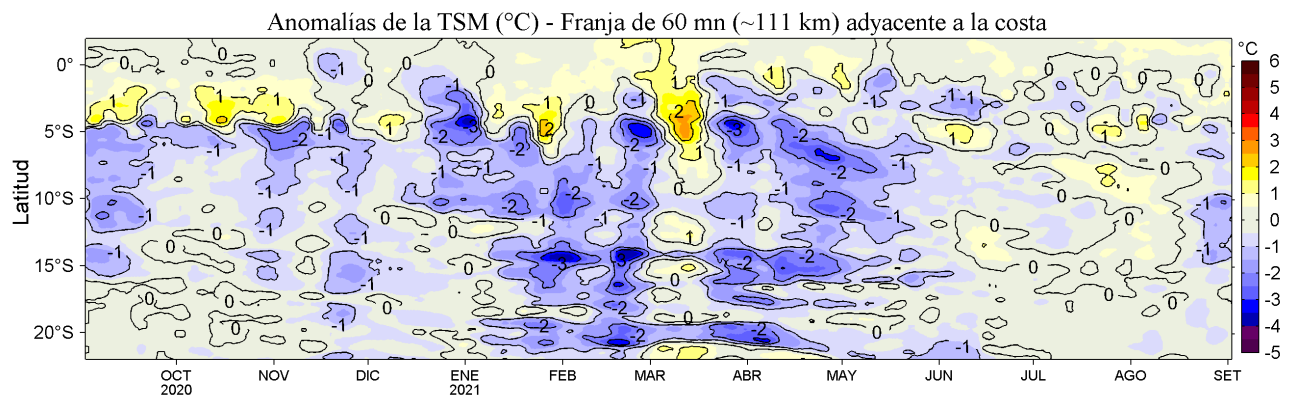
Figura 4. Variación promedio de las anomalías de la temperatura superficial del mar (TSM, °C) para una franja de 60 m.n. (~111 km) adyacente al litoral peruano para los últimos doce meses al 02 de setiembre de 2021. Datos: OSTIA-UKMO-L4-GLOB-v2.0 (UK Met. Office, 2012; Donlon et al, 2012) disponible en https://podaac.jpl.nasa.gov/dataset/OSTIA-UKMO-L4-GLOB-v2.0 . Las anomalías se calcularon con respecto al periodo 2007-2016.
