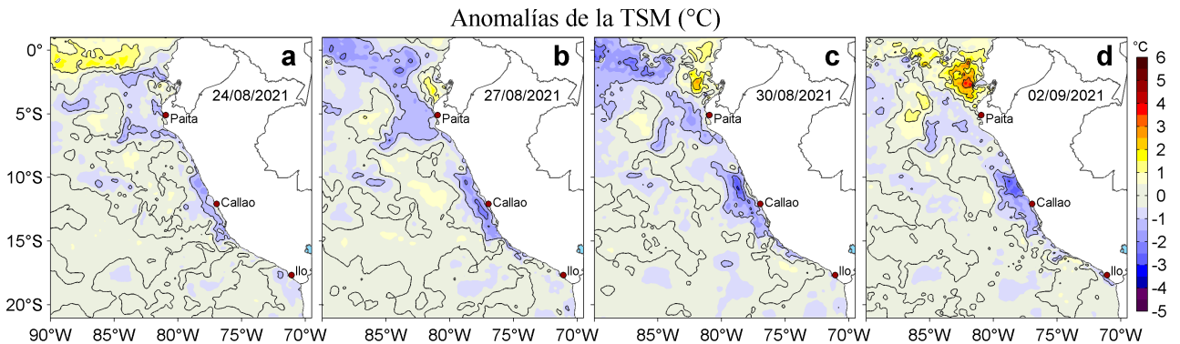
Figura 3. Anomalías de la temperatura superficial del mar (TSM, °C) para los días: a) 24, b) 27 y c) 30 de agosto y d) 02 de setiembre de 2021. Las anomalías se calcularon respecto de la climatología para el periodo 2007-2016. Datos: OSTIA-UKMO-L4-GLOB-v2.0 (UK Met Office, 2012; Donlon et al, 2012).
