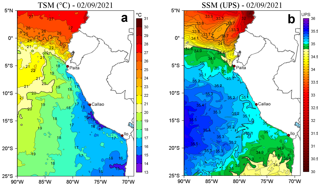
Figura 2. a) Temperatura superficial del mar (TSM, °C) y b) Salinidad superficial del mar (SSM) para el 02 de setiembre de 2021. Datos: OSTIA-UKMO-L4-GLOB-v2.0 (UK Met Office, 2012; Donlon et al, 2012) disponible en https://podaac.jpl.nasa.gov/dataset/OSTIA-UKMO-L4-GLOB-v2.0 para (a) y Hybrid Coordinate Ocean Model v. GOFS 3.1 (HYCOM; Halliwell et al., 1998; 2000; Bleck, 2001) para (b).
