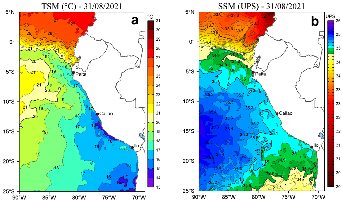
Figura 2. a) Temperatura superficial del mar (TSM, °C) y b) Salinidad superficial del mar (SSM) para el 31 de agosto de 2021. Datos: OSTIA-UKMO-L4-GLOB-v2.0 (UK Met Office, 2012; Donlon et al, 2012) disponible en https://podaac.jpl.nasa.gov/dataset/OSTIA-UKMO-L4-GLOB-v2.0 para (a) y Hybrid Coordinate Ocean Model v. GOFS 3.1 (HYCOM; Halliwell et al., 1998; 2000; Bleck, 2001) para (b).
