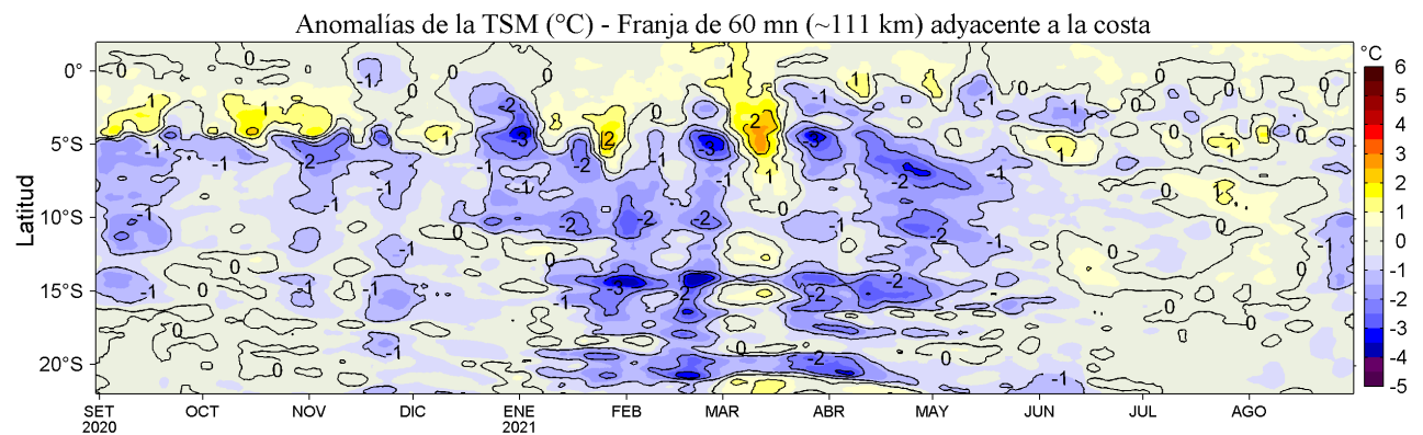
Figura 4. Variación promedio de las anomalías de la temperatura superficial del mar (TSM, °C) para una franja de 60 m.n. (~111 km) adyacente al litoral peruano para los últimos doce meses al 31 de agosto de 2021. Datos: OSTIA-UKMO-L4-GLOB-v2.0 (UK Met. Office, 2012; Donlon et al, 2012) disponible en https://podaac.jpl.nasa.gov/dataset/OSTIA-UKMO-L4-GLOB-v2.0 . Las anomalías se calcularon con respecto al periodo 2007-2016.
