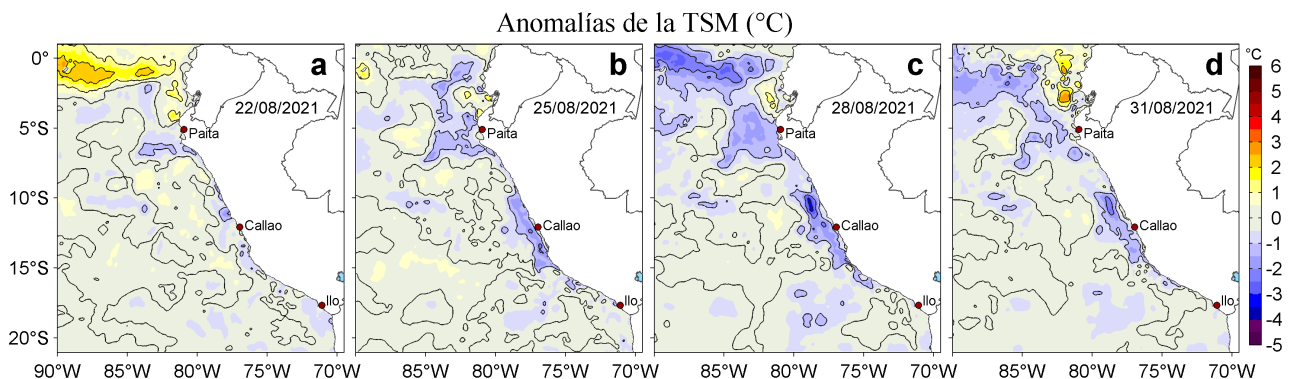
Figura 3. Anomalías de la temperatura superficial del mar (TSM, °C) para los días: a) 22, b) 25, c) 28 y d) 31 de agosto de 2021. Las anomalías se calcularon respecto de la climatología para el periodo 2007-2016. Datos: OSTIA-UKMO-L4-GLOB-v2.0 (UK Met Office, 2012; Donlon et al, 2012).
