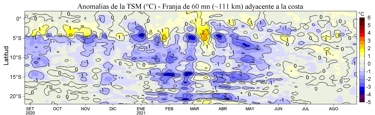
Figura 4. Variación promedio de las anomalías de la temperatura superficial del mar (TSM, °C) para una franja de 60 m.n. (~111 km) adyacente al litoral peruano para los últimos doce meses al 26 de agosto de 2021. Datos: OSTIA-UKMO-L4-GLOB-v2.0 (UK Met. Office, 2012; Donlon et al, 2012) disponible en https://podaac.jpl.nasa.gov/dataset/OSTIA-UKMO-L4-GLOB-v2.0 . Las anomalías se calcularon con respecto al periodo 2007-2016.
