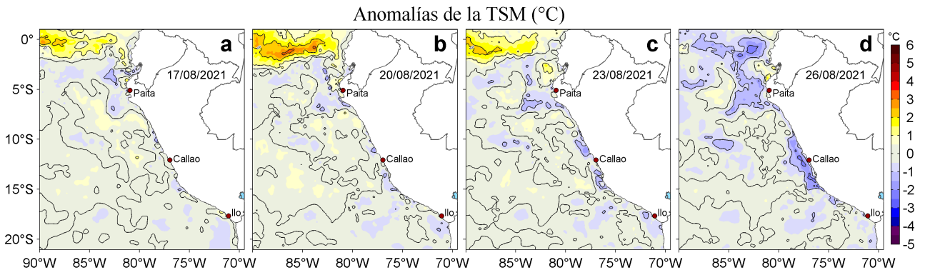
Figura 3. Anomalías de la temperatura superficial del mar (TSM, °C) para los días: a) 17, b) 20, c) 23 y d) 26 de agosto de 2021. Las anomalías se calcularon respecto de la climatología para el periodo 2007-2016. Datos: OSTIA-UKMO-L4-GLOB-v2.0 (UK Met Office, 2012; Donlon et al, 2012).
