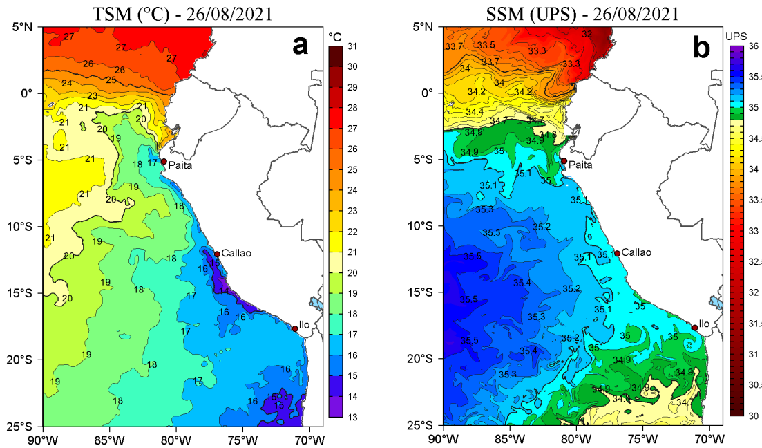
Figura 2. a) Temperatura superficial del mar (TSM, °C) y b) Salinidad superficial del mar (SSM) para el 26 de agosto de 2021. Datos: OSTIA-UKMO-L4-GLOB-v2.0 (UK Met Office, 2012; Donlon et al, 2012) disponible en https://podaac.jpl.nasa.gov/dataset/OSTIA-UKMO-L4-GLOB-v2.0 para (a) y Hybrid Coordinate Ocean Model v. GOFS 3.1 (HYCOM; Halliwell et al., 1998; 2000; Bleck, 2001) para (b).
