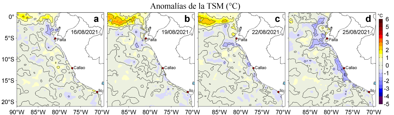
Figura 3. Anomalías de la temperatura superficial del mar (TSM, °C) para los días: a) 16, b) 19, c) 22 y d) 25 de agosto de 2021. Las anomalías se calcularon respecto de la climatología para el periodo 2007-2016. Datos: OSTIA-UKMO-L4-GLOB-v2.0 (UK Met Office, 2012; Donlon et al, 2012).
