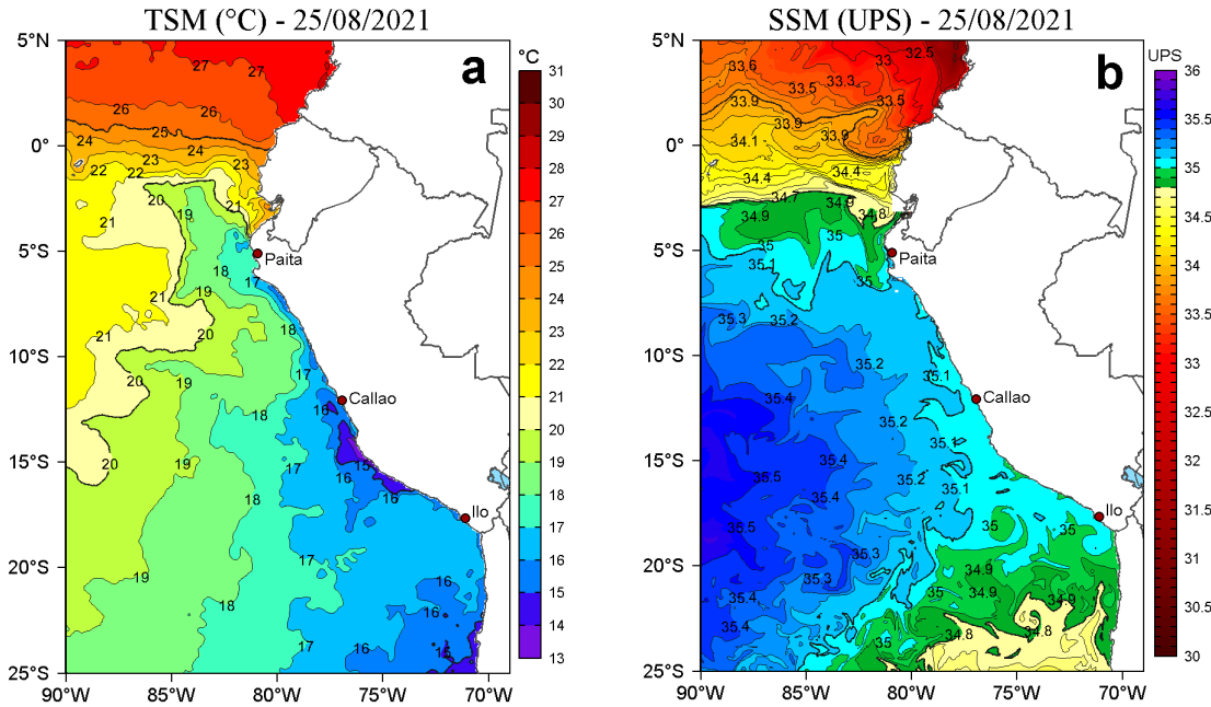
Figura 2. a) Temperatura superficial del mar (TSM, °C) y b) Salinidad superficial del mar (SSM) para el 25 de agosto de 2021. Datos: OSTIA-UKMO-L4-GLOB-v2.0 (UK Met Office, 2012; Donlon et al, 2012) disponible en https://podaac.jpl.nasa.gov/dataset/OSTIA-UKMO-L4-GLOB-v2.0 para (a) y Hybrid Coordinate Ocean Model v. GOFS 3.1 (HYCOM; Halliwell et al., 1998; 2000; Bleck, 2001) para (b).
