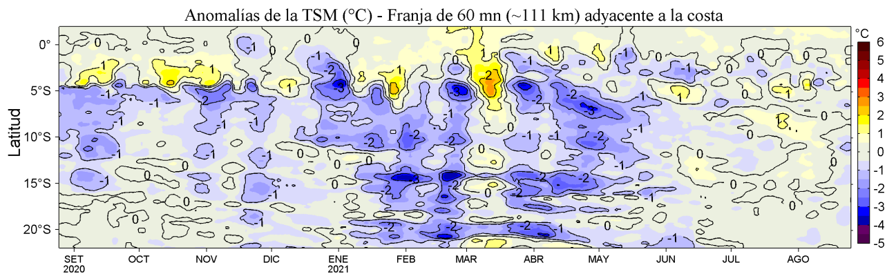
Figura 4. Variación promedio de las anomalías de la temperatura superficial del mar (TSM, °C) para una franja de 60 m.n. (~111 km) adyacente al litoral peruano para los últimos doce meses al 25 de agosto de 2021. Datos: OSTIA-UKMO-L4-GLOB-v2.0 (UK Met. Office, 2012; Donlon et al, 2012) disponible en https://podaac.jpl.nasa.gov/dataset/OSTIA-UKMO-L4-GLOB-v2.0 . Las anomalías se calcularon con respecto al periodo 2007-2016.
