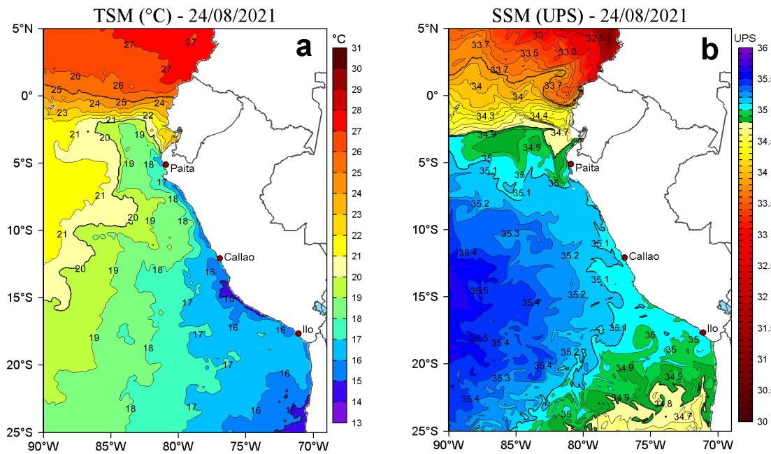
Figura 2. a) Temperatura superficial del mar (TSM, °C) y b) Salinidad superficial del mar (SSM) para el 24 de agosto de 2021. Datos: OSTIA-UKMO-L4-GLOB-v2.0 (UK Met Office, 2012; Donlon et al, 2012) disponible en https://podaac.jpl.nasa.gov/dataset/OSTIA-UKMO-L4-GLOB-v2.0 para (a) y Hybrid Coordinate Ocean Model v. GOFS 3.1 (HYCOM; Halliwell et al., 1998; 2000; Bleck, 2001) para (b).
