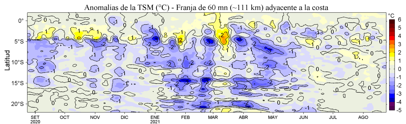
Figura 4. Variación promedio de las anomalías de la temperatura superficial del mar (TSM, °C) para una franja de 60 m.n. (~111 km) adyacente al litoral peruano para los últimos doce meses al 24 de agosto de 2021. Datos: OSTIA-UKMO-L4-GLOB-v2.0 (UK Met. Office, 2012; Donlon et al, 2012) disponible en https://podaac.jpl.nasa.gov/dataset/OSTIA-UKMO-L4-GLOB-v2.0 . Las anomalías se calcularon con respecto al periodo 2007-2016.
