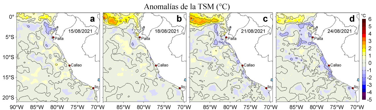
Figura 3. Anomalías de la temperatura superficial del mar (TSM, °C) para los días: a) 15, b) 18, c) 21 y d) 24 de agosto de 2021. Las anomalías se calcularon respecto de la climatología para el periodo 2007-2016. Datos: OSTIA-UKMO-L4-GLOB-v2.0 (UK Met Office, 2012; Donlon et al, 2012).
