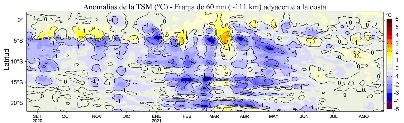
Figura 4. Variación promedio de las anomalías de la temperatura superficial del mar (TSM, °C) para una franja de 60 m.n. (~111 km) adyacente al litoral peruano para los últimos doce meses al 21 de agosto de 2021. Datos: OSTIA-UKMO-L4-GLOB-v2.0 (UK Met. Office, 2012; Donlon et al, 2012) disponible en https://podaac.jpl.nasa.gov/dataset/OSTIA-UKMO-L4-GLOB-v2.0 . Las anomalías se calcularon con respecto al periodo 2007-2016.
