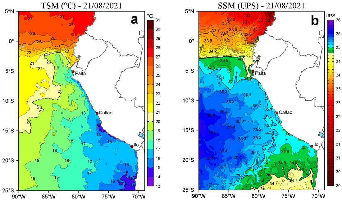
Figura 2. a) Temperatura superficial del mar (TSM, °C) y b) Salinidad superficial del mar (SSM) para el 21 de agosto de 2021. Datos: OSTIA-UKMO-L4-GLOB-v2.0 (UK Met Office, 2012; Donlon et al, 2012) disponible en https://podaac.jpl.nasa.gov/dataset/OSTIA-UKMO-L4-GLOB-v2.0 para (a) y Hybrid Coordinate Ocean Model v. GOFS 3.1 (HYCOM; Halliwell et al., 1998; 2000; Bleck, 2001) para (b).
