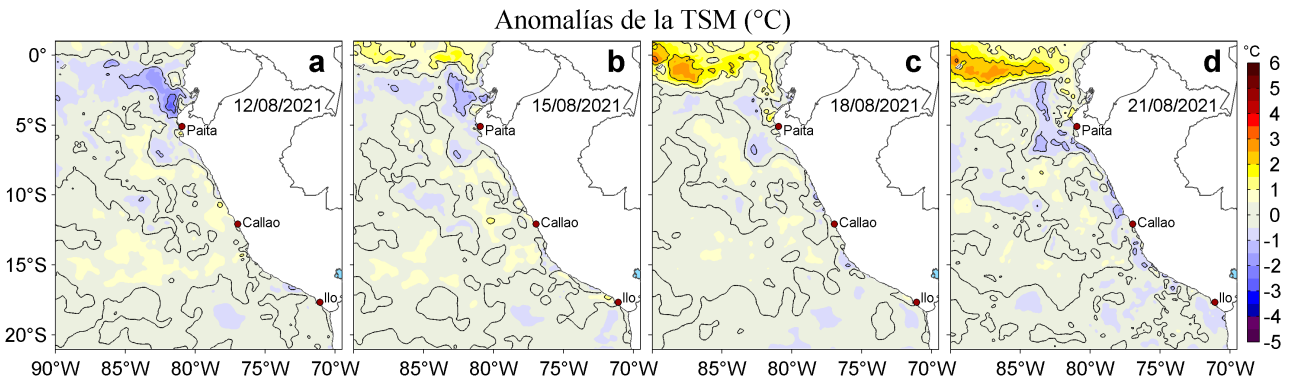
Figura 3. Anomalías de la temperatura superficial del mar (TSM, °C) para los días: a) 12, b) 15, c) 18 y d) 21 de agosto de 2021. Las anomalías se calcularon respecto de la climatología para el periodo 2007-2016. Datos: OSTIA-UKMO-L4-GLOB-v2.0 (UK Met Office, 2012; Donlon et al, 2012).
