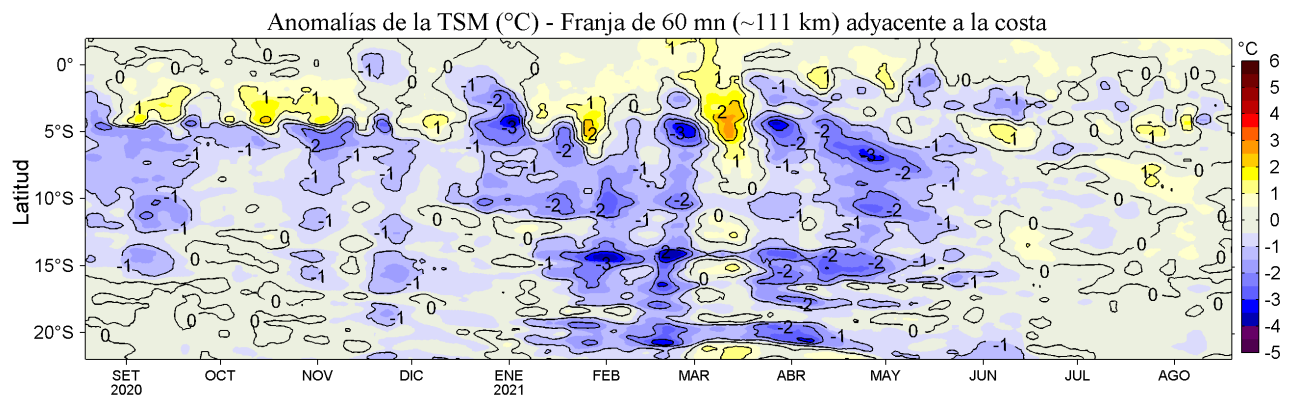
Figura 4. Variación promedio de las anomalías de la temperatura superficial del mar (TSM, °C) para una franja de 60 m.n. (~111 km) adyacente al litoral peruano para los últimos doce meses al 19 de agosto de 2021. Datos: OSTIA-UKMO-L4-GLOB-v2.0 (UK Met. Office, 2012; Donlon et al, 2012) disponible en https://podaac.jpl.nasa.gov/dataset/OSTIA-UKMO-L4-GLOB-v2.0 . Las anomalías se calcularon con respecto al periodo 2007-2016.
