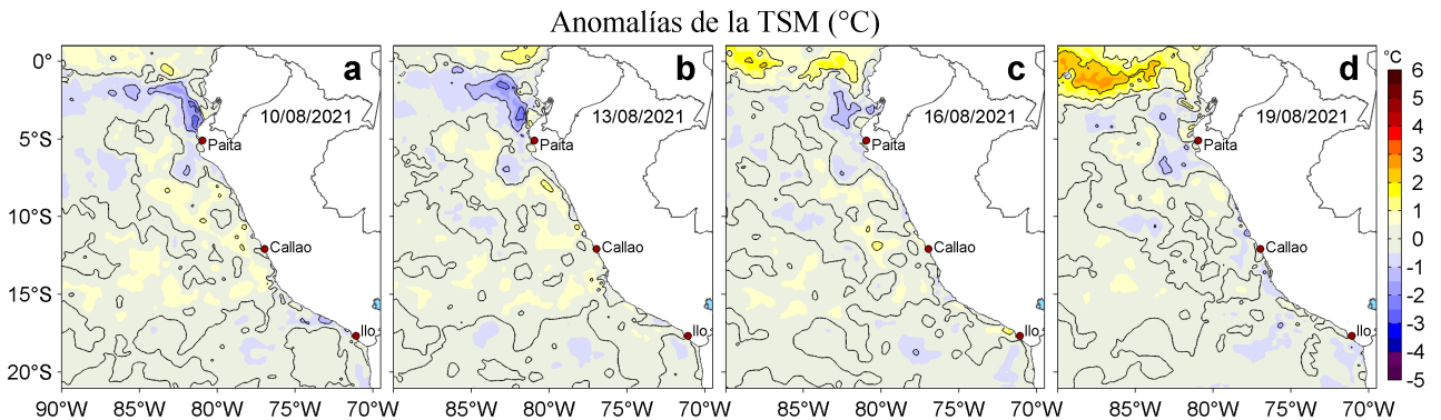
Figura 3. Anomalías de la temperatura superficial del mar (TSM, °C) para los días: a) 10, b) 13, c) 16 y d) 19 de agosto de 2021. Las anomalías se calcularon respecto de la climatología para el periodo 2007-2016. Datos: OSTIA-UKMO-L4-GLOB-v2.0 (UK Met Office, 2012; Donlon et al, 2012).
