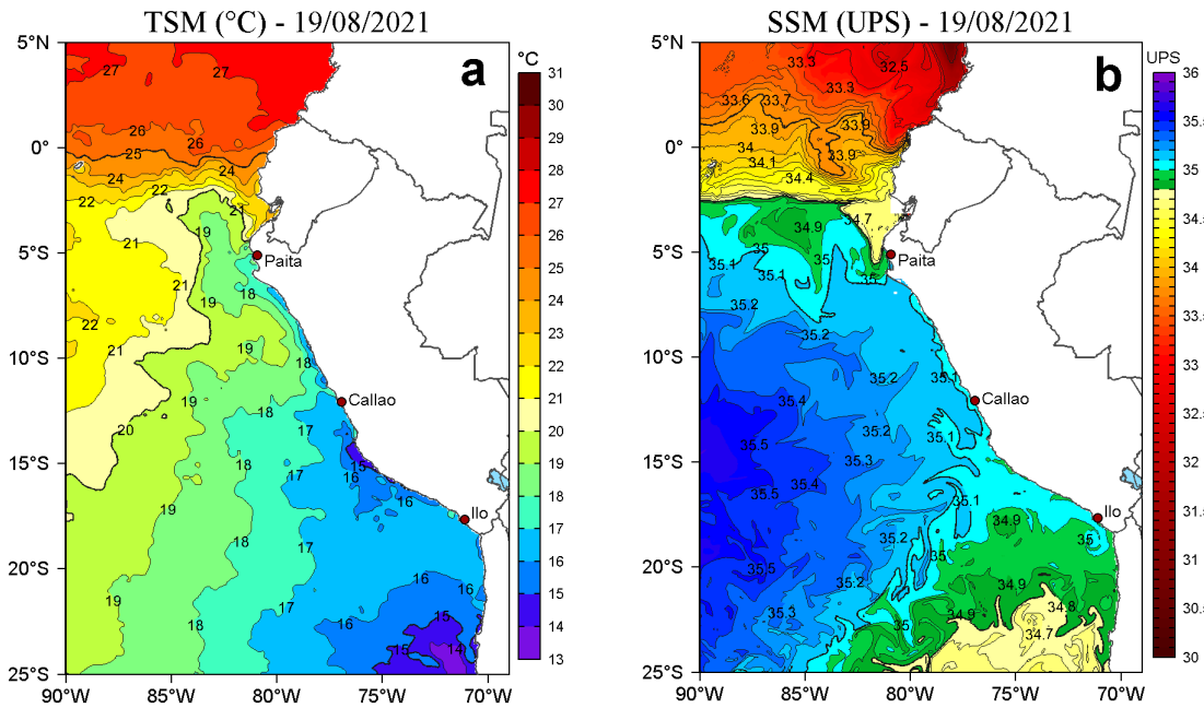
Figura 2. a) Temperatura superficial del mar (TSM, °C) y b) Salinidad superficial del mar (SSM) para el 19 de agosto de 2021. Datos: OSTIA-UKMO-L4-GLOB-v2.0 (UK Met Office, 2012; Donlon et al, 2012) disponible en https://podaac.jpl.nasa.gov/dataset/OSTIA-UKMO-L4-GLOB-v2.0 para (a) y Hybrid Coordinate Ocean Model v. GOFS 3.1 (HYCOM; Halliwell et al., 1998; 2000; Bleck, 2001) para (b).
