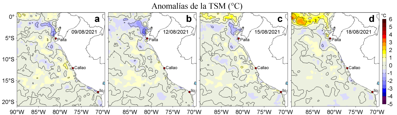
Figura 3. Anomalías de la temperatura superficial del mar (TSM, °C) para los días: a) 09, b) 12, c) 15 y d) 18 de agosto de 2021. Las anomalías se calcularon respecto de la climatología para el periodo 2007-2016. Datos: OSTIA-UKMO-L4-GLOB-v2.0 (UK Met Office, 2012; Donlon et al, 2012).
