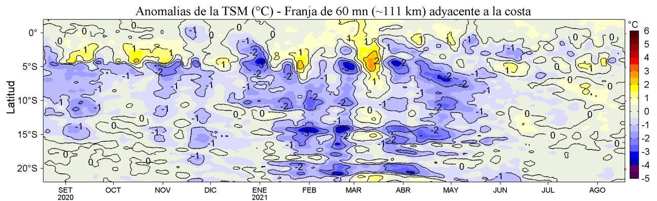
Figura 4. Variación promedio de las anomalías de la temperatura superficial del mar (TSM, °C) para una franja de 60 m.n. (~111 km) adyacente al litoral peruano para los últimos doce meses al 18 de agosto de 2021. Datos: OSTIA-UKMO-L4-GLOB-v2.0 (UK Met. Office, 2012; Donlon et al, 2012) disponible en https://podaac.jpl.nasa.gov/dataset/OSTIA-UKMO-L4-GLOB-v2.0 . Las anomalías se calcularon con respecto al periodo 2007-2016.
