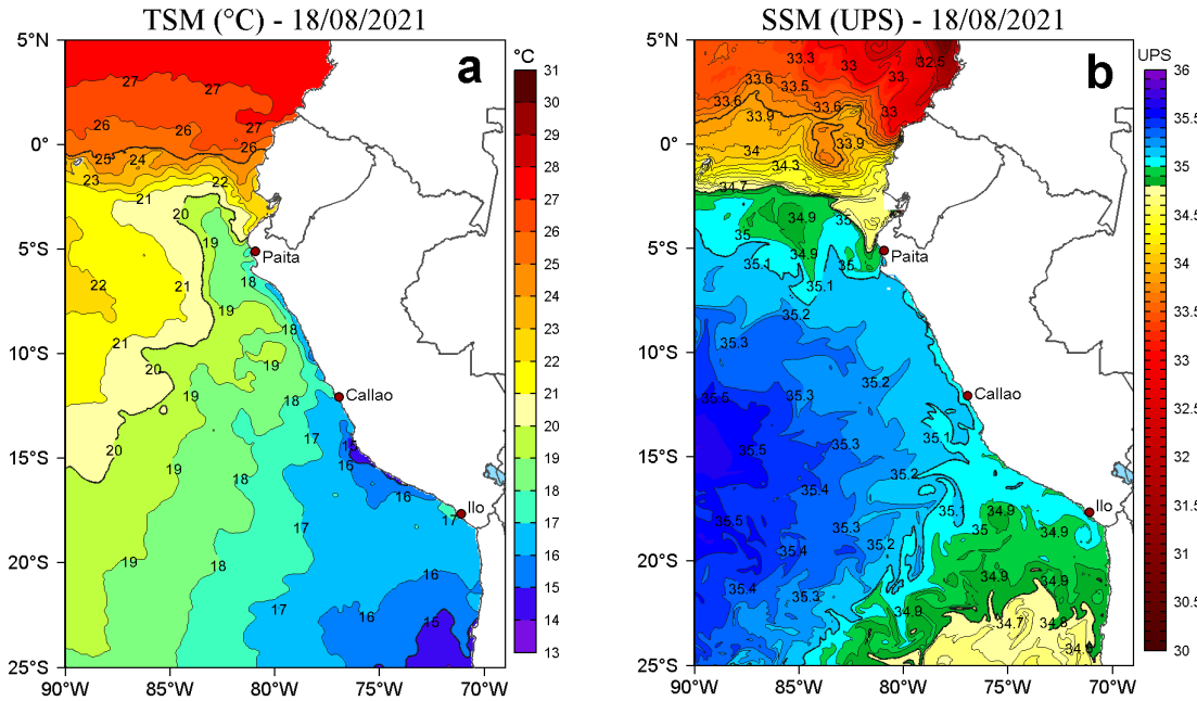
Figura 2. a) Temperatura superficial del mar (TSM, °C) y b) Salinidad superficial del mar (SSM) para el 18 de agosto de 2021. Datos: OSTIA-UKMO-L4-GLOB-v2.0 (UK Met Office, 2012; Donlon et al, 2012) disponible en https://podaac.jpl.nasa.gov/dataset/OSTIA-UKMO-L4-GLOB-v2.0 para (a) y Hybrid Coordinate Ocean Model v. GOFS 3.1 (HYCOM; Halliwell et al., 1998; 2000; Bleck, 2001) para (b).
