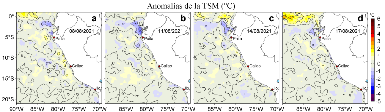
Figura 3. Anomalías de la temperatura superficial del mar (TSM, °C) para los días: a) 08, b) 11, c) 14 y d) 17 de agosto de 2021. Las anomalías se calcularon respecto de la climatología para el periodo 2007-2016. Datos: OSTIA-UKMO-L4-GLOB-v2.0 (UK Met Office, 2012; Donlon et al, 2012).
