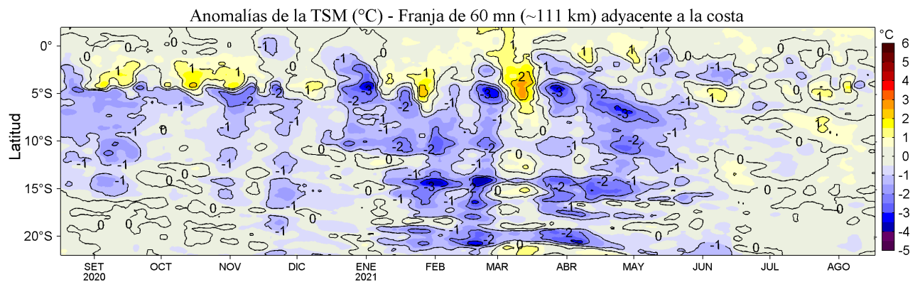
Figura 4. Variación promedio de las anomalías de la temperatura superficial del mar (TSM, °C) para una franja de 60 m.n. (~111 km) adyacente al litoral peruano para los últimos doce meses al 17 de agosto de 2021. Datos: OSTIA-UKMO-L4-GLOB-v2.0 (UK Met. Office, 2012; Donlon et al, 2012) disponible en https://podaac.jpl.nasa.gov/dataset/OSTIA-UKMO-L4-GLOB-v2.0 . Las anomalías se calcularon con respecto al periodo 2007-2016.
