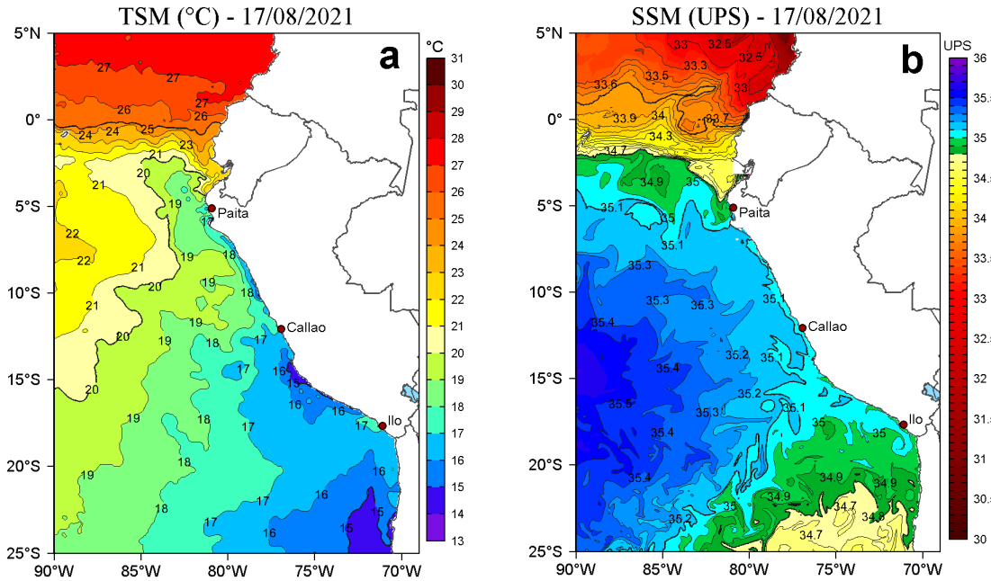
Figura 2. a) Temperatura superficial del mar (TSM, °C) y b) Salinidad superficial del mar (SSM) para el 17 de agosto de 2021. Datos: OSTIA-UKMO-L4-GLOB-v2.0 (UK Met Office, 2012; Donlon et al, 2012) disponible en https://podaac.jpl.nasa.gov/dataset/OSTIA-UKMO-L4-GLOB-v2.0 para (a) y Hybrid Coordinate Ocean Model v. GOFS 3.1 (HYCOM; Halliwell et al., 1998; 2000; Bleck, 2001) para (b).
