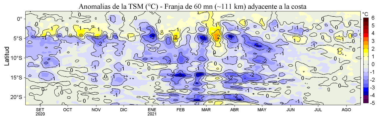
Figura 4. Variación promedio de las anomalías de la temperatura superficial del mar (TSM, °C) para una franja de 60 m.n. (~111 km) adyacente al litoral peruano para los últimos doce meses al 16 de agosto de 2021. Datos: OSTIA-UKMO-L4-GLOB-v2.0 (UK Met. Office, 2012; Donlon et al, 2012) disponible en https://podaac.jpl.nasa.gov/dataset/OSTIA-UKMO-L4-GLOB-v2.0 . Las anomalías se calcularon con respecto al periodo 2007-2016.
