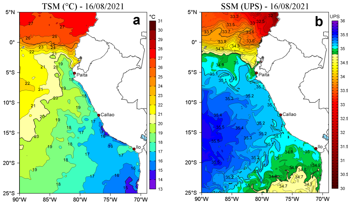
Figura 2. a) Temperatura superficial del mar (TSM, °C) y b) Salinidad superficial del mar (SSM) para el 16 de agosto de 2021. Datos: OSTIA-UKMO-L4-GLOB-v2.0 (UK Met Office, 2012; Donlon et al, 2012) disponible en https://podaac.jpl.nasa.gov/dataset/OSTIA-UKMO-L4-GLOB-v2.0 para (a) y Hybrid Coordinate Ocean Model v. GOFS 3.1 (HYCOM; Halliwell et al., 1998; 2000; Bleck, 2001) para (b).
