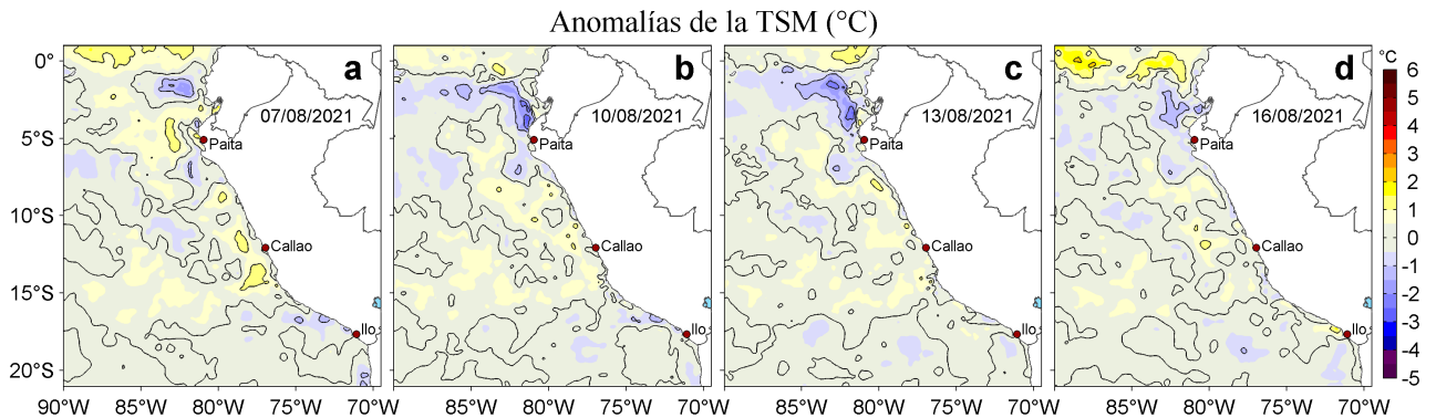
Figura 3. Anomalías de la temperatura superficial del mar (TSM, °C) para los días: a) 07, b) 10, c) 13 y d) 16 de agosto de 2021. Las anomalías se calcularon respecto de la climatología para el periodo 2007-2016. Datos: OSTIA-UKMO-L4-GLOB-v2.0 (UK Met Office, 2012; Donlon et al, 2012).
