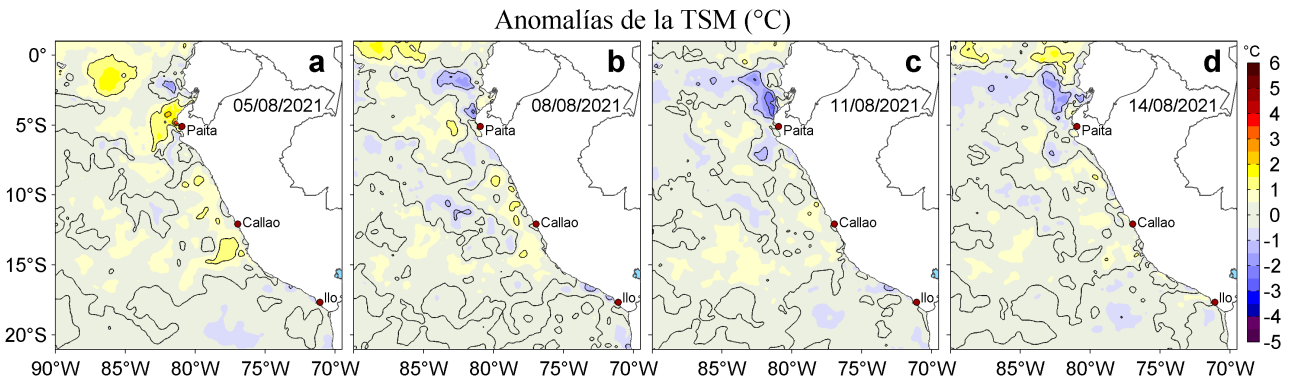
Figura 3. Anomalías de la temperatura superficial del mar (TSM, °C) para los días: a) 05, b) 08, c) 11 y d) 14 de agosto de 2021. Las anomalías se calcularon respecto de la climatología para el periodo 2007-2016. Datos: OSTIA-UKMO-L4-GLOB-v2.0 (UK Met Office, 2012; Donlon et al, 2012).
