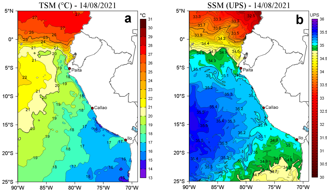
Figura 2. a) Temperatura superficial del mar (TSM, °C) y b) Salinidad superficial del mar (SSM) para el 14 de agosto de 2021. Datos: OSTIA-UKMO-L4-GLOB-v2.0 (UK Met Office, 2012; Donlon et al, 2012) disponible en https://podaac.jpl.nasa.gov/dataset/OSTIA-UKMO-L4-GLOB-v2.0 para (a) y Hybrid Coordinate Ocean Model v. GOFS 3.1 (HYCOM; Halliwell et al., 1998; 2000; Bleck, 2001) para (b).
