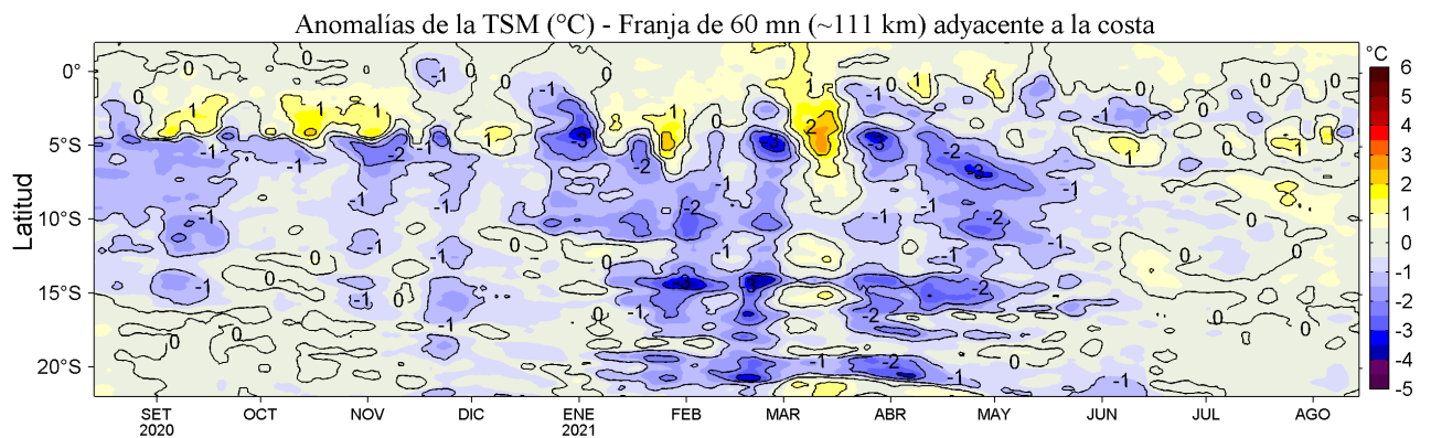
Figura 4. Variación promedio de las anomalías de la temperatura superficial del mar (TSM, °C) para una franja de 60 m.n. (~111 km) adyacente al litoral peruano para los últimos doce meses al 14 de agosto de 2021. Datos: OSTIA-UKMO-L4-GLOB-v2.0 (UK Met. Office, 2012; Donlon et al, 2012) disponible en https://podaac.jpl.nasa.gov/dataset/OSTIA-UKMO-L4-GLOB-v2.0 . Las anomalías se calcularon con respecto al periodo 2007-2016.
