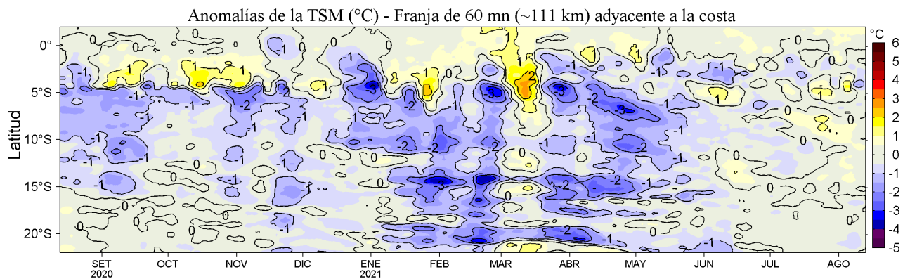
Figura 4. Variación promedio de las anomalías de la temperatura superficial del mar (TSM, °C) para una franja de 60 m.n. (~111 km) adyacente al litoral peruano para los últimos doce meses al 13 de agosto de 2021. Datos: OSTIA-UKMO-L4-GLOB-v2.0 (UK Met. Office, 2012; Donlon et al, 2012) disponible en https://podaac.jpl.nasa.gov/dataset/OSTIA-UKMO-L4-GLOB-v2.0 . Las anomalías se calcularon con respecto al periodo 2007-2016.
