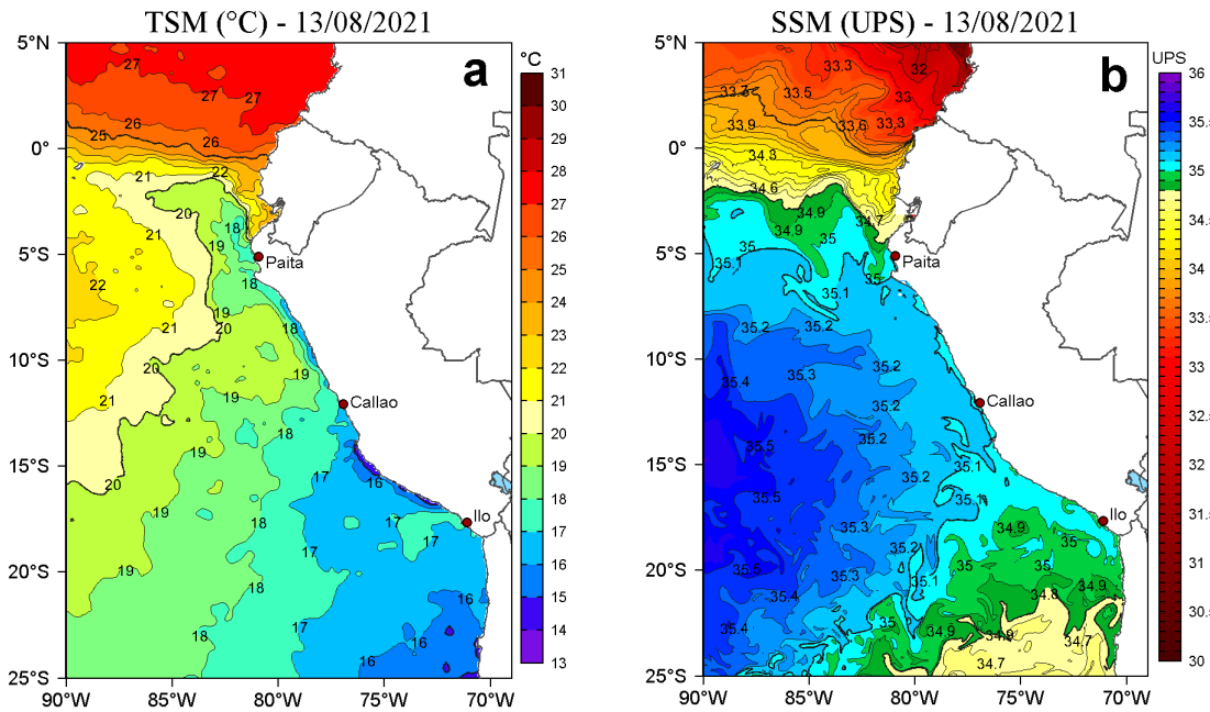
Figura 2. a) Temperatura superficial del mar (TSM, °C) y b) Salinidad superficial del mar (SSM) para el 13 de agosto de 2021. Datos: OSTIA-UKMO-L4-GLOB-v2.0 (UK Met Office, 2012; Donlon et al, 2012) disponible en https://podaac.jpl.nasa.gov/dataset/OSTIA-UKMO-L4-GLOB-v2.0 para (a) y Hybrid Coordinate Ocean Model v. GOFS 3.1 (HYCOM; Halliwell et al., 1998; 2000; Bleck, 2001) para (b).
