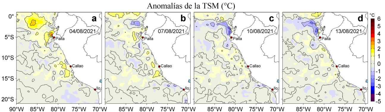
Figura 3. Anomalías de la temperatura superficial del mar (TSM, °C) para los días: a) 04, b) 07, c) 10 y d) 13 de agosto de 2021. Las anomalías se calcularon respecto de la climatología para el periodo 2007-2016. Datos: OSTIA-UKMO-L4-GLOB-v2.0 (UK Met Office, 2012; Donlon et al, 2012).
