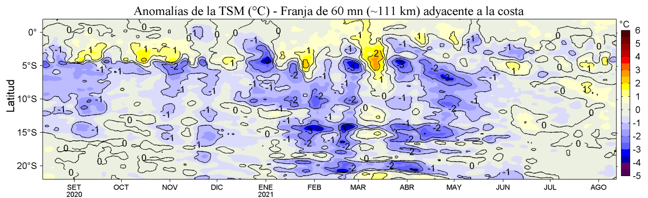
Figura 4. Variación promedio de las anomalías de la temperatura superficial del mar (TSM, °C) para una franja de 60 m.n. (~111 km) adyacente al litoral peruano para los últimos doce meses al 12 de agosto de 2021. Datos: OSTIA-UKMO-L4-GLOB-v2.0 (UK Met. Office, 2012; Donlon et al, 2012) disponible en https://podaac.jpl.nasa.gov/dataset/OSTIA-UKMO-L4-GLOB-v2.0 . Las anomalías se calcularon con respecto al periodo 2007-2016.
