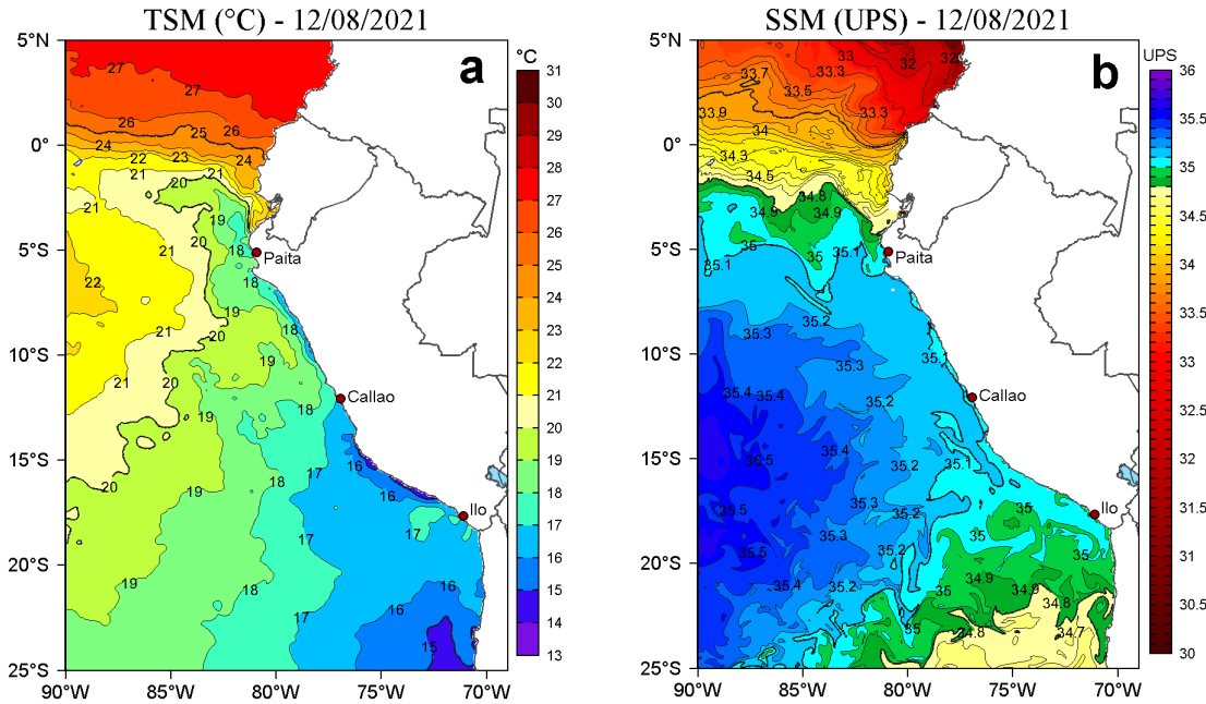
Figura 2. a) Temperatura superficial del mar (TSM, °C) y b) Salinidad superficial del mar (SSM) para el 12 de agosto de 2021. Datos: OSTIA-UKMO-L4-GLOB-v2.0 (UK Met Office, 2012; Donlon et al, 2012) disponible en https://podaac.jpl.nasa.gov/dataset/OSTIA-UKMO-L4-GLOB-v2.0 para (a) y Hybrid Coordinate Ocean Model v. GOFS 3.1 (HYCOM; Halliwell et al., 1998; 2000; Bleck, 2001) para (b).
