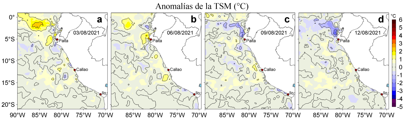
Figura 3. Anomalías de la temperatura superficial del mar (TSM, °C) para los días: a) 03, b) 06, c) 09 y d) 12 de agosto de 2021. Las anomalías se calcularon respecto de la climatología para el periodo 2007-2016. Datos: OSTIA-UKMO-L4-GLOB-v2.0 (UK Met Office, 2012; Donlon et al, 2012).
