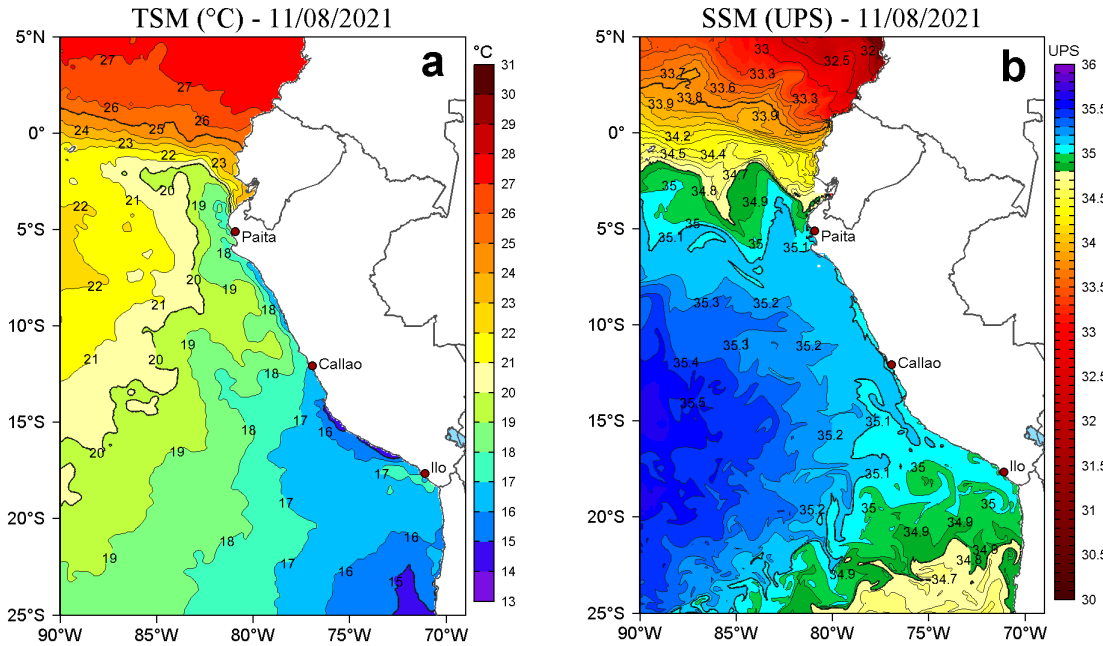
Figura 2. a) Temperatura superficial del mar (TSM, °C) y b) Salinidad superficial del mar (SSM) para el 11 de agosto de 2021. Datos: OSTIA-UKMO-L4-GLOB-v2.0 (UK Met Office, 2012; Donlon et al, 2012) disponible en https://podaac.jpl.nasa.gov/dataset/OSTIA-UKMO-L4-GLOB-v2.0 para (a) y Hybrid Coordinate Ocean Model v. GOFS 3.1 (HYCOM; Halliwell et al., 1998; 2000; Bleck, 2001) para (b).
