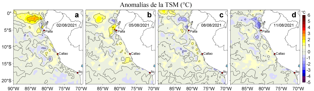
Figura 3. Anomalías de la temperatura superficial del mar (TSM, °C) para los días: a) 02, b) 05, c) 08 y d) 11 de agosto de 2021. Las anomalías se calcularon respecto de la climatología para el periodo 2007-2016. Datos: OSTIA-UKMO-L4-GLOB-v2.0 (UK Met Office, 2012; Donlon et al, 2012).
