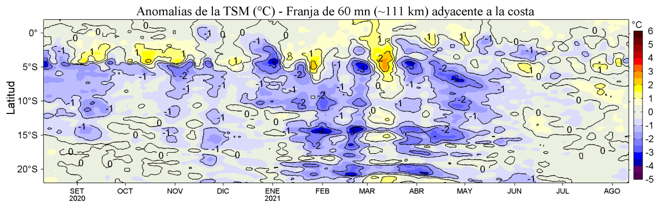
Figura 4. Variación promedio de las anomalías de la temperatura superficial del mar (TSM, °C) para una franja de 60 m.n. (~111 km) adyacente al litoral peruano para los últimos doce meses al 11 de agosto de 2021. Datos: OSTIA-UKMO-L4-GLOB-v2.0 (UK Met. Office, 2012; Donlon et al, 2012) disponible en https://podaac.jpl.nasa.gov/dataset/OSTIA-UKMO-L4-GLOB-v2.0 . Las anomalías se calcularon con respecto al periodo 2007-2016.
