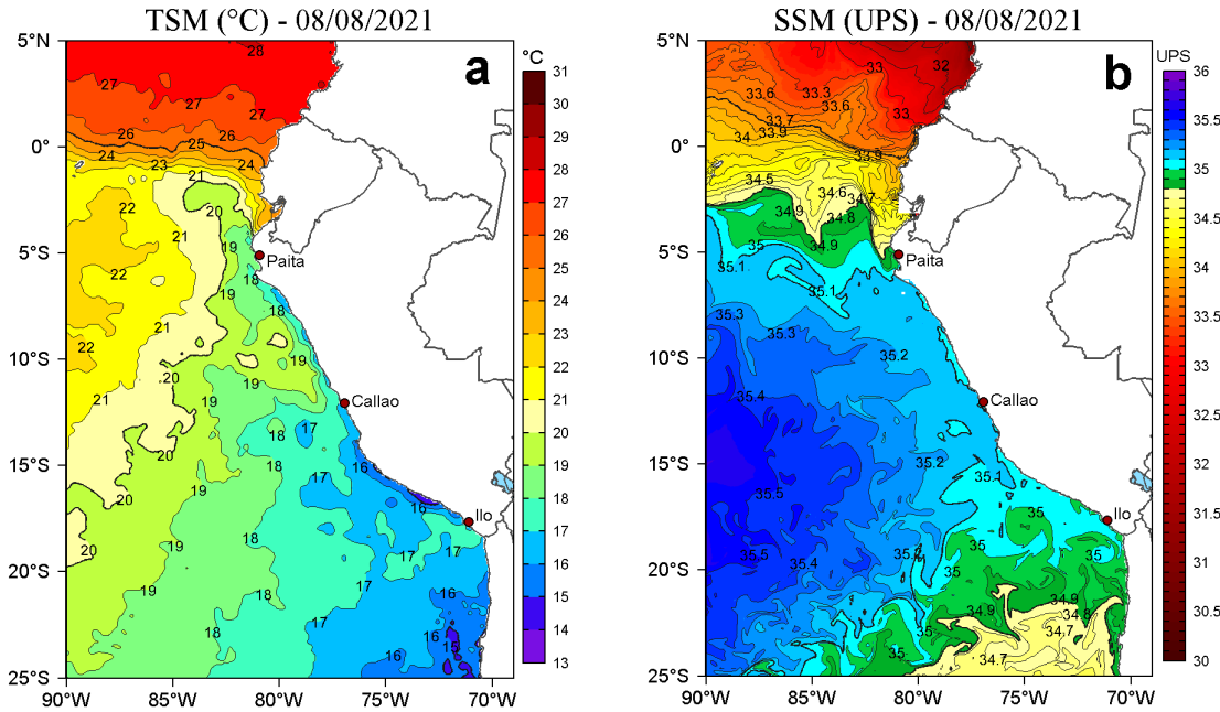
Figura 2. a) Temperatura superficial del mar (TSM, °C) y b) Salinidad superficial del mar (SSM) para el 08 de agosto de 2021. Datos: OSTIA-UKMO-L4-GLOB-v2.0 (UK Met Office, 2012; Donlon et al, 2012) disponible en https://podaac.jpl.nasa.gov/dataset/OSTIA-UKMO-L4-GLOB-v2.0 para (a) y Hybrid Coordinate Ocean Model v. GOFS 3.1 (HYCOM; Halliwell et al., 1998; 2000; Bleck, 2001) para (b).
