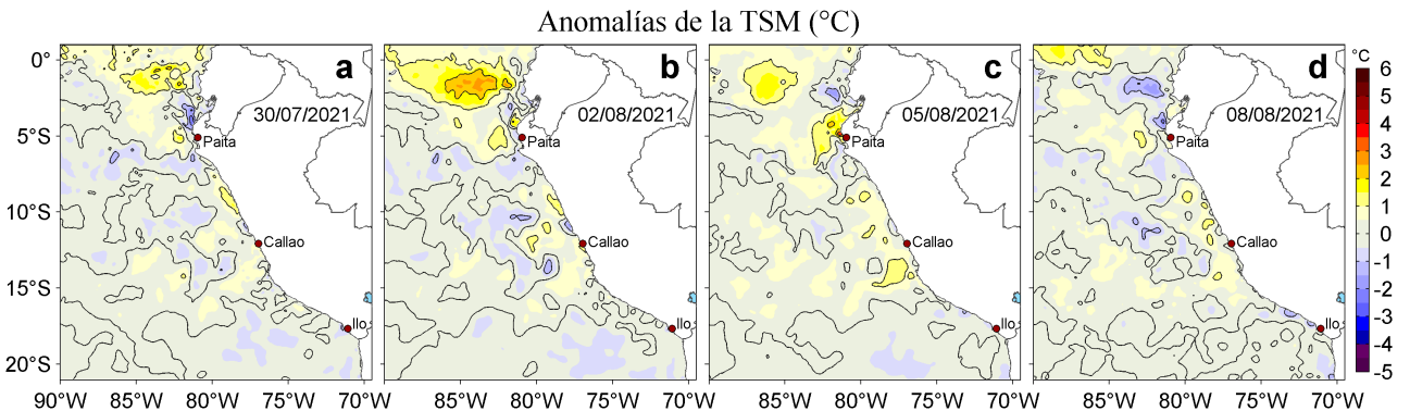
Figura 3. Anomalías de la temperatura superficial del mar (TSM, °C) para los días: a) 30 de julio, b) 02, c) 05 y d) 08 de agosto de 2021. Las anomalías se calcularon respecto de la climatología para el periodo 2007-2016. Datos: OSTIA-UKMO-L4-GLOB-v2.0 (UK Met Office, 2012; Donlon et al, 2012).
