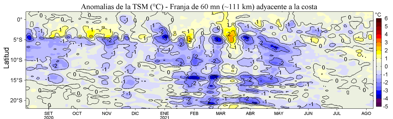
Figura 4. Variación promedio de las anomalías de la temperatura superficial del mar (TSM, °C) para una franja de 60 m.n. (~111 km) adyacente al litoral peruano para los últimos doce meses al 08 de agosto de 2021. Datos: OSTIA-UKMO-L4-GLOB-v2.0 (UK Met. Office, 2012; Donlon et al, 2012) disponible en https://podaac.jpl.nasa.gov/dataset/OSTIA-UKMO-L4-GLOB-v2.0 . Las anomalías se calcularon con respecto al periodo 2007-2016.
