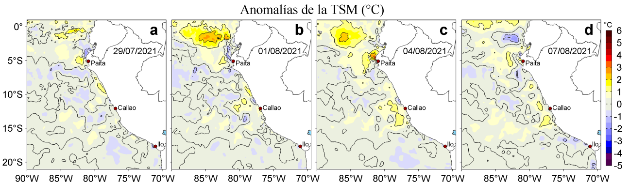
Figura 3. Anomalías de la temperatura superficial del mar (TSM, °C) para los días: a) 29 de julio, b) 01, c) 04 y d) 07 de agosto de 2021. Las anomalías se calcularon respecto de la climatología para el periodo 2007-2016. Datos: OSTIA-UKMO-L4-GLOB-v2.0 (UK Met Office, 2012; Donlon et al, 2012).
