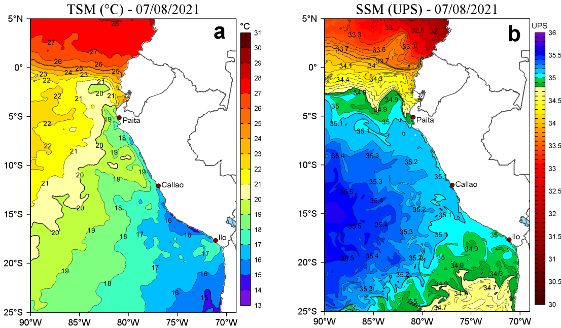
Figura 2. a) Temperatura superficial del mar (TSM, °C) y b) Salinidad superficial del mar (SSM) para el 07 de agosto de 2021. Datos: OSTIA-UKMO-L4-GLOB-v2.0 (UK Met Office, 2012; Donlon et al, 2012) disponible en https://podaac.jpl.nasa.gov/dataset/OSTIA-UKMO-L4-GLOB-v2.0 para (a) y Hybrid Coordinate Ocean Model v. GOFS 3.1 (HYCOM; Halliwell et al., 1998; 2000; Bleck, 2001) para (b).
