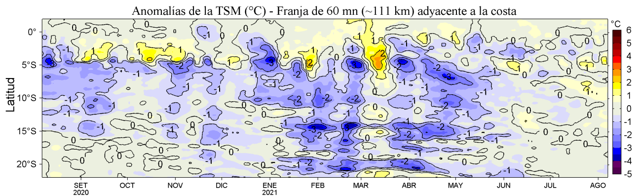
Figura 4. Variación promedio de las anomalías de la temperatura superficial del mar (TSM, °C) para una franja de 60 m.n. (~111 km) adyacente al litoral peruano para los últimos doce meses al 07 de agosto de 2021. Datos: OSTIA-UKMO-L4-GLOB-v2.0 (UK Met. Office, 2012; Donlon et al, 2012) disponible en https://podaac.jpl.nasa.gov/dataset/OSTIA-UKMO-L4-GLOB-v2.0 . Las anomalías se calcularon con respecto al periodo 2007-2016.
