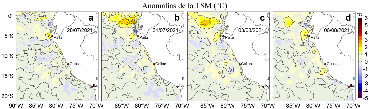
Figura 3. Anomalías de la temperatura superficial del mar (TSM, °C) para los días: a) 28 y b) 31 de julio, c) 03 y d) 06 de agosto de 2021. Las anomalías se calcularon respecto de la climatología para el periodo 2007-2016. Datos: OSTIA-UKMO-L4-GLOB-v2.0 (UK Met Office, 2012; Donlon et al, 2012).
