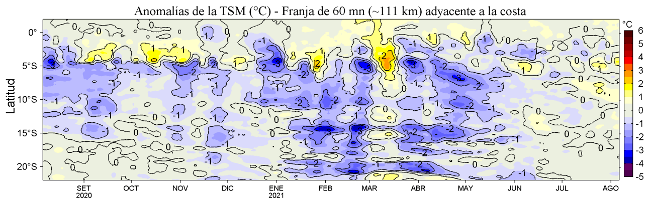
Figura 4. Variación promedio de las anomalías de la temperatura superficial del mar (TSM, °C) para una franja de 60 m.n. (~111 km) adyacente al litoral peruano para los últimos doce meses al 06 de agosto de 2021. Datos: OSTIA-UKMO-L4-GLOB-v2.0 (UK Met. Office, 2012; Donlon et al, 2012) disponible en https://podaac.jpl.nasa.gov/dataset/OSTIA-UKMO-L4-GLOB-v2.0 . Las anomalías se calcularon con respecto al periodo 2007-2016.
