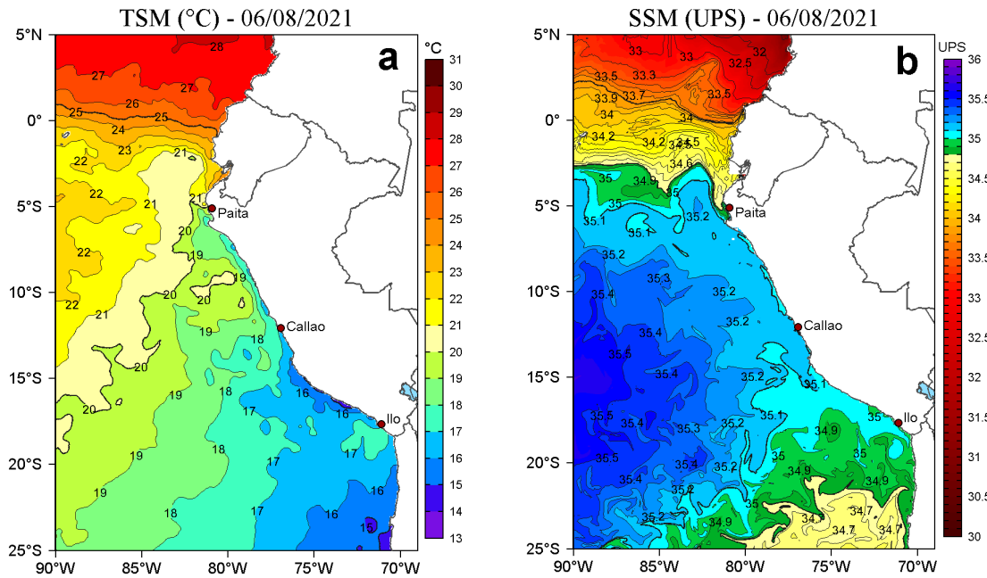
Figura 2. a) Temperatura superficial del mar (TSM, °C) y b) Salinidad superficial del mar (SSM) para el 06 de agosto de 2021. Datos: OSTIA-UKMO-L4-GLOB-v2.0 (UK Met Office, 2012; Donlon et al, 2012) disponible en https://podaac.jpl.nasa.gov/dataset/OSTIA-UKMO-L4-GLOB-v2.0 para (a) y Hybrid Coordinate Ocean Model v. GOFS 3.1 (HYCOM; Halliwell et al., 1998; 2000; Bleck, 2001) para (b).
