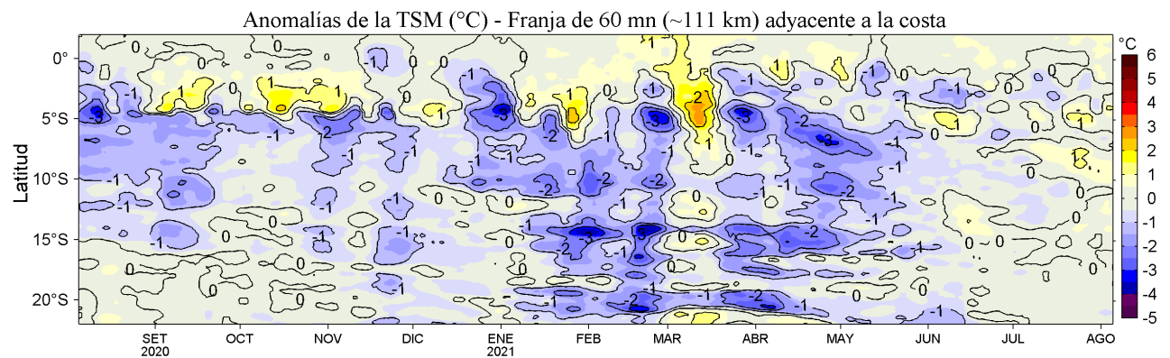
Figura 4. Variación promedio de las anomalías de la temperatura superficial del mar (TSM, °C) para una franja de 60 m.n. (~111 km) adyacente al litoral peruano para los últimos doce meses al 05 de agosto de 2021. Datos: OSTIA-UKMO-L4-GLOB-v2.0 (UK Met. Office, 2012; Donlon et al, 2012) disponible en https://podaac.jpl.nasa.gov/dataset/OSTIA-UKMO-L4-GLOB-v2.0 . Las anomalías se calcularon con respecto al periodo 2007-2016.
