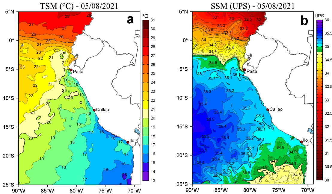
Figura 2. a) Temperatura superficial del mar (TSM, °C) y b) Salinidad superficial del mar (SSM) para el 05 de agosto de 2021. Datos: OSTIA-UKMO-L4-GLOB-v2.0 (UK Met Office, 2012; Donlon et al, 2012) disponible en https://podaac.jpl.nasa.gov/dataset/OSTIA-UKMO-L4-GLOB-v2.0 para (a) y Hybrid Coordinate Ocean Model v. GOFS 3.1 (HYCOM; Halliwell et al., 1998; 2000; Bleck, 2001) para (b).
