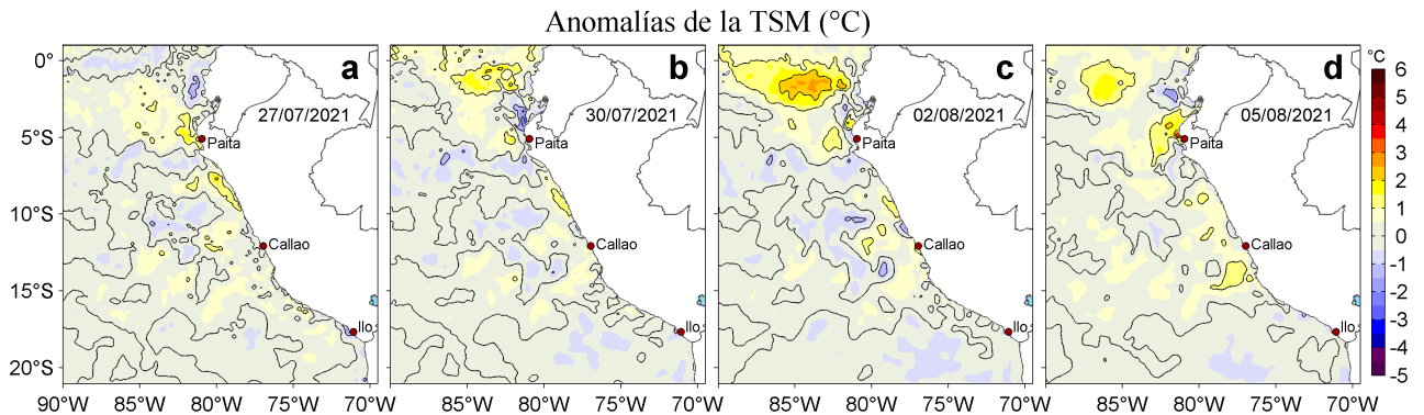
Figura 3. Anomalías de la temperatura superficial del mar (TSM, °C) para los días: a) 27 y b) 30 de julio, c) 02 y d) 05 de agosto de 2021. Las anomalías se calcularon respecto de la climatología para el periodo 2007-2016. Datos: OSTIA-UKMO-L4-GLOB-v2.0 (UK Met Office, 2012; Donlon et al, 2012).
