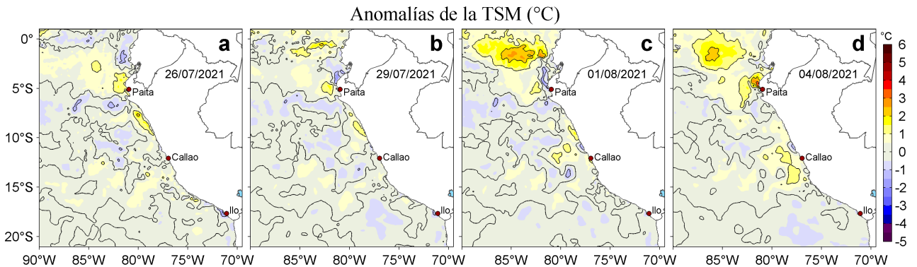
Figura 3. Anomalías de la temperatura superficial del mar (TSM, °C) para los días: a) 26 y b) 29 de julio, c) 01 y d) 04 de agosto de 2021. Las anomalías se calcularon respecto de la climatología para el periodo 2007-2016. Datos: OSTIA-UKMO-L4-GLOB-v2.0 (UK Met Office, 2012; Donlon et al, 2012).
