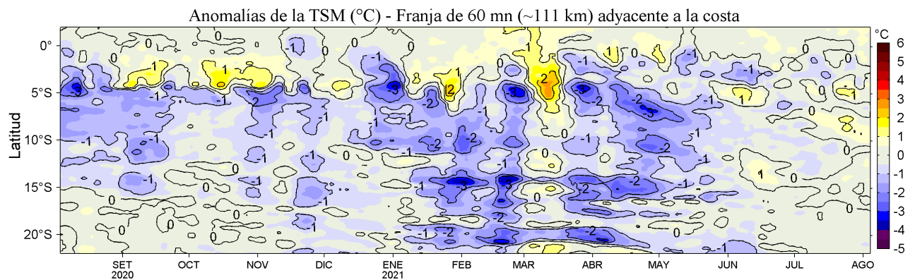
Figura 4. Variación promedio de las anomalías de la temperatura superficial del mar (TSM, °C) para una franja de 60 m.n. (~111 km) adyacente al litoral peruano para los últimos doce meses al 04 de agosto de 2021. Datos: OSTIA-UKMO-L4-GLOB-v2.0 (UK Met. Office, 2012; Donlon et al, 2012) disponible en https://podaac.jpl.nasa.gov/dataset/OSTIA-UKMO-L4-GLOB-v2.0 . Las anomalías se calcularon con respecto al periodo 2007-2016.
