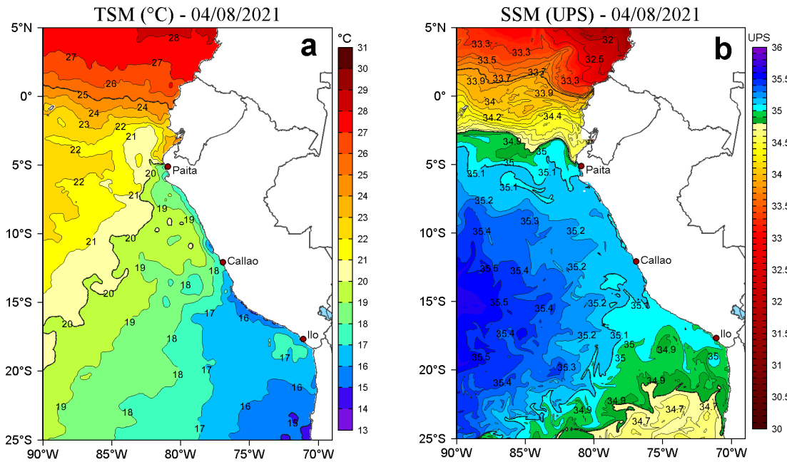
Figura 2. a) Temperatura superficial del mar (TSM, °C) y b) Salinidad superficial del mar (SSM) para el 04 de agosto de 2021. Datos: OSTIA-UKMO-L4-GLOB-v2.0 (UK Met Office, 2012; Donlon et al, 2012) disponible en https://podaac.jpl.nasa.gov/dataset/OSTIA-UKMO-L4-GLOB-v2.0 para (a) y Hybrid Coordinate Ocean Model v. GOFS 3.1 (HYCOM; Halliwell et al., 1998; 2000; Bleck, 2001) para (b).
