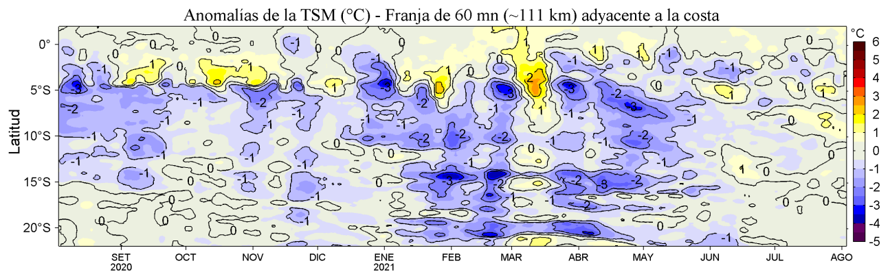
Figura 4. Variación promedio de las anomalías de la temperatura superficial del mar (TSM, °C) para una franja de 60 m.n. (~111 km) adyacente al litoral peruano para los últimos doce meses al 03 de agosto de 2021. Datos: OSTIA-UKMO-L4-GLOB-v2.0 (UK Met. Office, 2012; Donlon et al, 2012) disponible en https://podaac.jpl.nasa.gov/dataset/OSTIA-UKMO-L4-GLOB-v2.0 . Las anomalías se calcularon con respecto al periodo 2007-2016.
