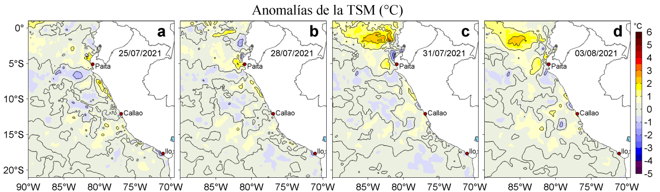
Figura 3. Anomalías de la temperatura superficial del mar (TSM, °C) para los días: a) 25, b) 28 y c) 31 de julio y d) 03 de agosto de 2021. Las anomalías se calcularon respecto de la climatología para el periodo 2007-2016. Datos: OSTIA-UKMO-L4-GLOB-v2.0 (UK Met Office, 2012; Donlon et al, 2012).
