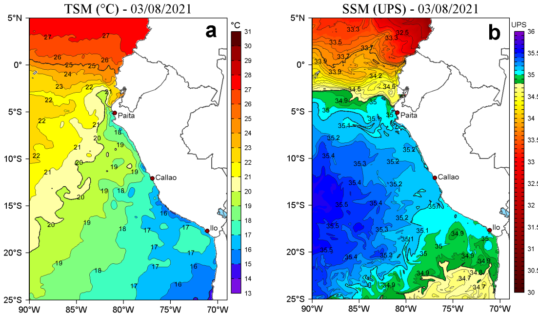
Figura 2. a) Temperatura superficial del mar (TSM, °C) y b) Salinidad superficial del mar (SSM) para el 03 de agosto de 2021. Datos: OSTIA-UKMO-L4-GLOB-v2.0 (UK Met Office, 2012; Donlon et al, 2012) disponible en https://podaac.jpl.nasa.gov/dataset/OSTIA-UKMO-L4-GLOB-v2.0 para (a) y Hybrid Coordinate Ocean Model v. GOFS 3.1 (HYCOM; Halliwell et al., 1998; 2000; Bleck, 2001) para (b).
