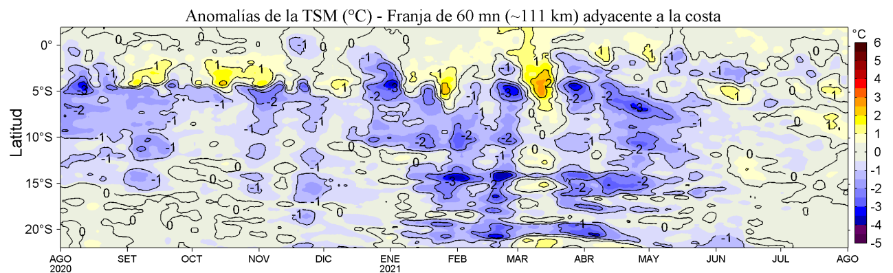
Figura 4. Variación promedio de las anomalías de la temperatura superficial del mar (TSM, °C) para una franja de 60 m.n. (~111 km) adyacente al litoral peruano para los últimos doce meses al 01 de agosto de 2021. Datos: OSTIA-UKMO-L4-GLOB-v2.0 (UK Met. Office, 2012; Donlon et al, 2012) disponible en https://podaac.jpl.nasa.gov/dataset/OSTIA-UKMO-L4-GLOB-v2.0 . Las anomalías se calcularon con respecto al periodo 2007-2016.
