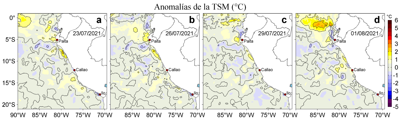
Figura 3. Anomalías de la temperatura superficial del mar (TSM, °C) para los días: a) 23, b) 26 y c) 29 de julio y d) 01 de agosto de 2021. Las anomalías se calcularon respecto de la climatología para el periodo 2007-2016. Datos: OSTIA-UKMO-L4-GLOB-v2.0 (UK Met Office, 2012; Donlon et al, 2012).
