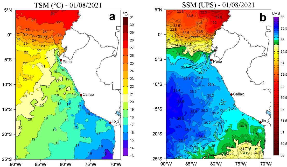
Figura 2. a) Temperatura superficial del mar (TSM, °C) y b) Salinidad superficial del mar (SSM) para el 01 de agosto de 2021. Datos: OSTIA-UKMO-L4-GLOB-v2.0 (UK Met Office, 2012; Donlon et al, 2012) disponible en https://podaac.jpl.nasa.gov/dataset/OSTIA-UKMO-L4-GLOB-v2.0 para (a) y Hybrid Coordinate Ocean Model v. GOF5 3.1 (HYCOM; Halliwell et al., 1998; 2000; Bleck, 2001) para (b).
