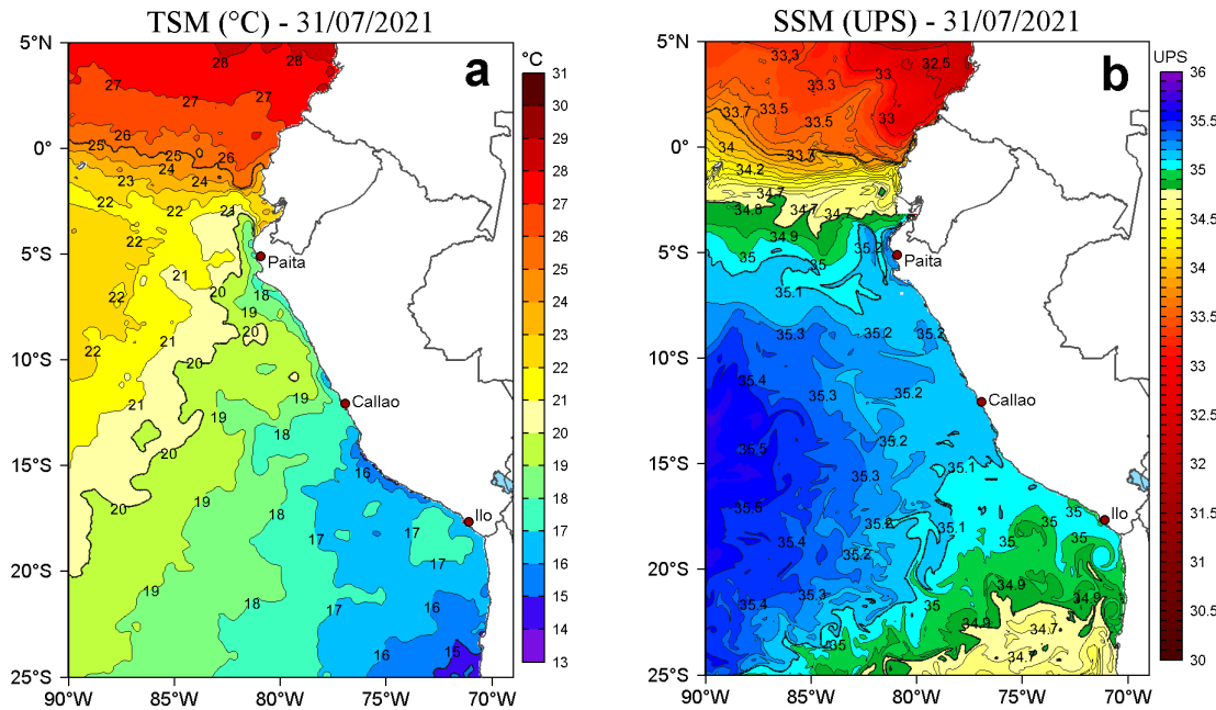
Figura 2. a) Temperatura superficial del mar (TSM, °C) y b) Salinidad superficial del mar (SSM) para el 31 de julio de 2021. Datos: OSTIA-UKMO-L4-GLOB-v2.0 (UK Met Office, 2012; Donlon et al, 2012) disponible en https://podaac.jpl.nasa.gov/dataset/OSTIA-UKMO-L4-GLOB-v2.0 para (a) y Hybrid Coordinate Ocean Model v. GOFS 3.1 (HYCOM; Halliwell et al., 1998; 2000; Bleck, 2001) para (b).
