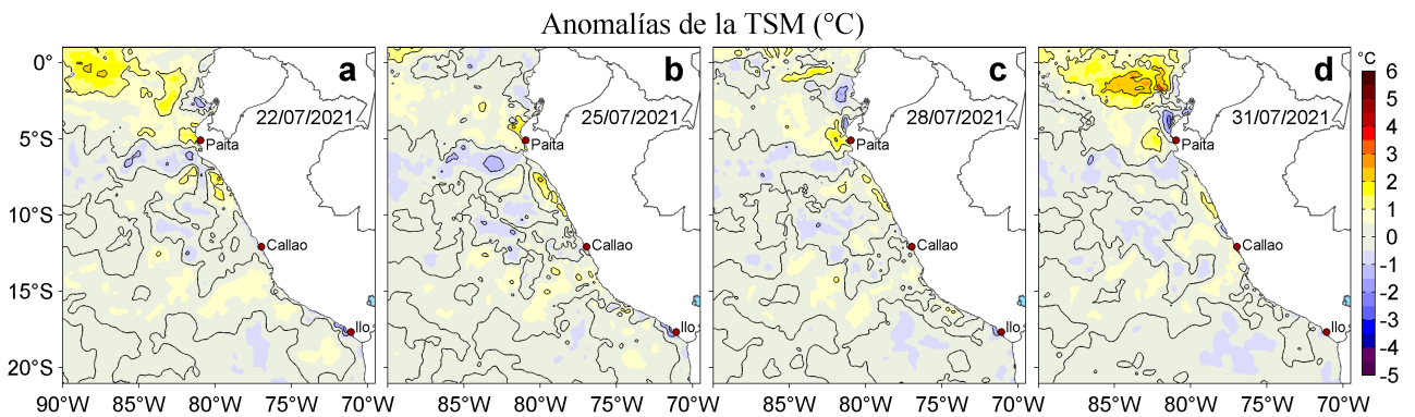
Figura 3. Anomalías de la temperatura superficial del mar (TSM, °C) para los días: a) 22, b) 25, c) 28 y d) 31 de julio de 2021. Las anomalías se calcularon respecto de la climatología para el periodo 2007-2016. Datos: OSTIA-UKMO-L4-GLOB-v2.0 (UK Met Office, 2012; Donlon et al, 2012).
