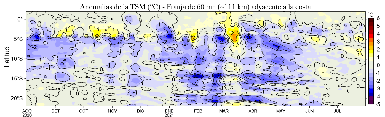
Figura 4. Variación promedio de las anomalías de la temperatura superficial del mar (TSM, °C) para una franja de 60 m.n. (~111 km) adyacente al litoral peruano para los últimos doce meses al 31 de julio de 2021. Datos: OSTIA-UKMO-L4-GLOB-v2.0 (UK Met. Office, 2012; Donlon et al, 2012) disponible en https://podaac.jpl.nasa.gov/dataset/OSTIA-UKMO-L4-GLOB-v2.0 . Las anomalías se calcularon con respecto al periodo 2007-2016.
