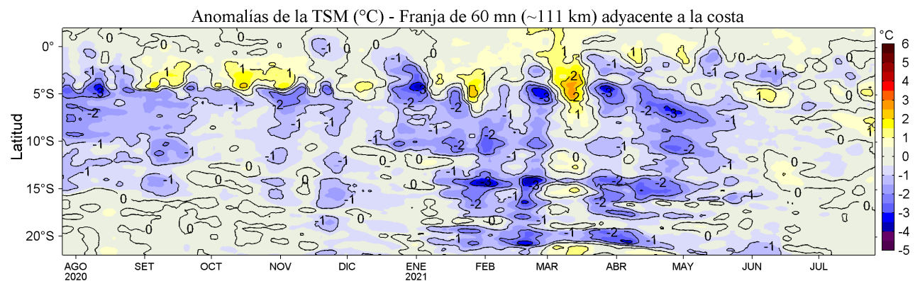
Figura 4. Variación promedio de las anomalías de la temperatura superficial del mar (TSM, °C) para una franja de 60 m.n. (~111 km) adyacente al litoral peruano para los últimos doce meses al 26 de julio de 2021. Datos: OSTIA-UKMO-L4-GLOB-v2.0 (UK Met. Office, 2012; Donlon et al, 2012) disponible en https://podaac.jpl.nasa.gov/dataset/OSTIA-UKMO-L4-GLOB-v2.0 . Las anomalías se calcularon con respecto al periodo 2007-2016.
