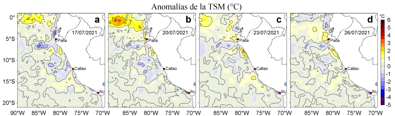
Figura 3. Anomalías de la temperatura superficial del mar (TSM, °C) para los días: a) 17, b) 20, c) 23 y d) 26 de julio de 2021. Las anomalías se calcularon respecto de la climatología para el periodo 2007-2016. Datos: OSTIA-UKMO-L4-GLOB-v2.0 (UK Met Office, 2012; Donlon et al, 2012).
