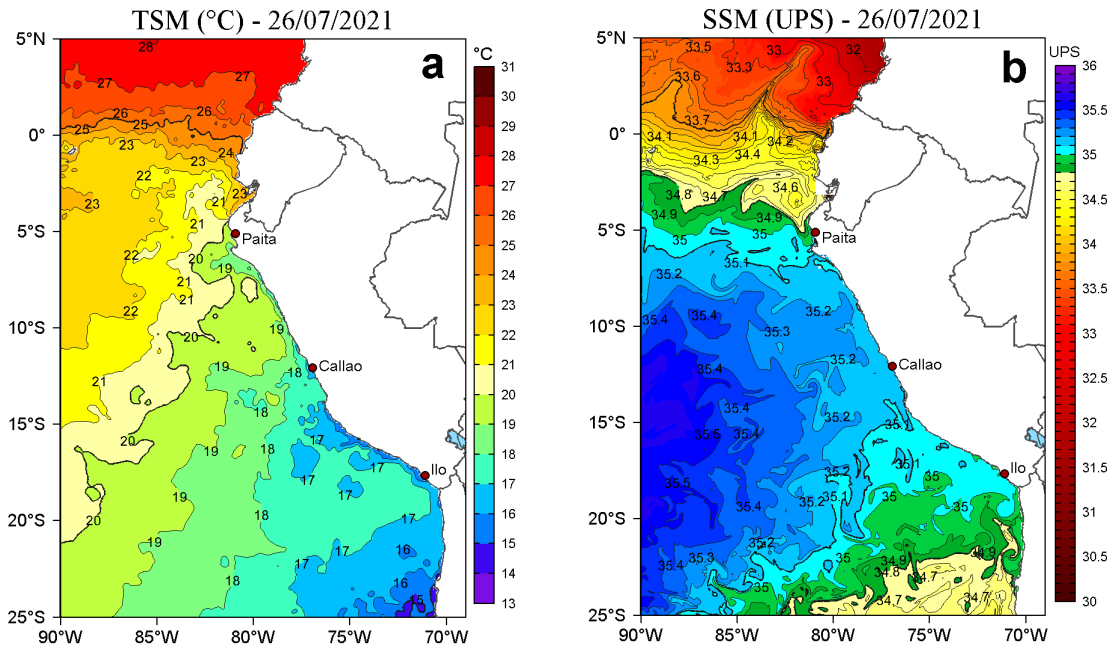
Figura 2. a) Temperatura superficial del mar (TSM, °C) y b) Salinidad superficial del mar (SSM) para el 26 de julio de 2021. Datos: OSTIA-UKMO-L4-GLOB-v2.0 (UK Met Office, 2012; Donlon et al, 2012) disponible en https://podaac.jpl.nasa.gov/dataset/OSTIA-UKMO-L4-GLOB-v2.0 para (a) y Hybrid Coordinate Ocean Model v. GOF5 3.1 (HYCOM; Halliwell et al., 1998; 2000; Bleck, 2001) para (b).
