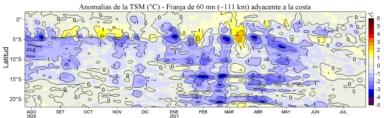
Figura 4. Variación promedio de las anomalías de la temperatura superficial del mar (TSM, °C) para una franja de 60 m.n. (~111 km) adyacente al litoral peruano para los últimos doce meses al 25 de julio de 2021. Datos: OSTIA-UKMO-L4-GLOB-v2.0 (UK Met. Office, 2012; Donlon et al, 2012) disponible en https://podaac.jpl.nasa.gov/dataset/OSTIA-UKMO-L4-GLOB-v2.0 . Las anomalías se calcularon con respecto al periodo 2007-2016.
