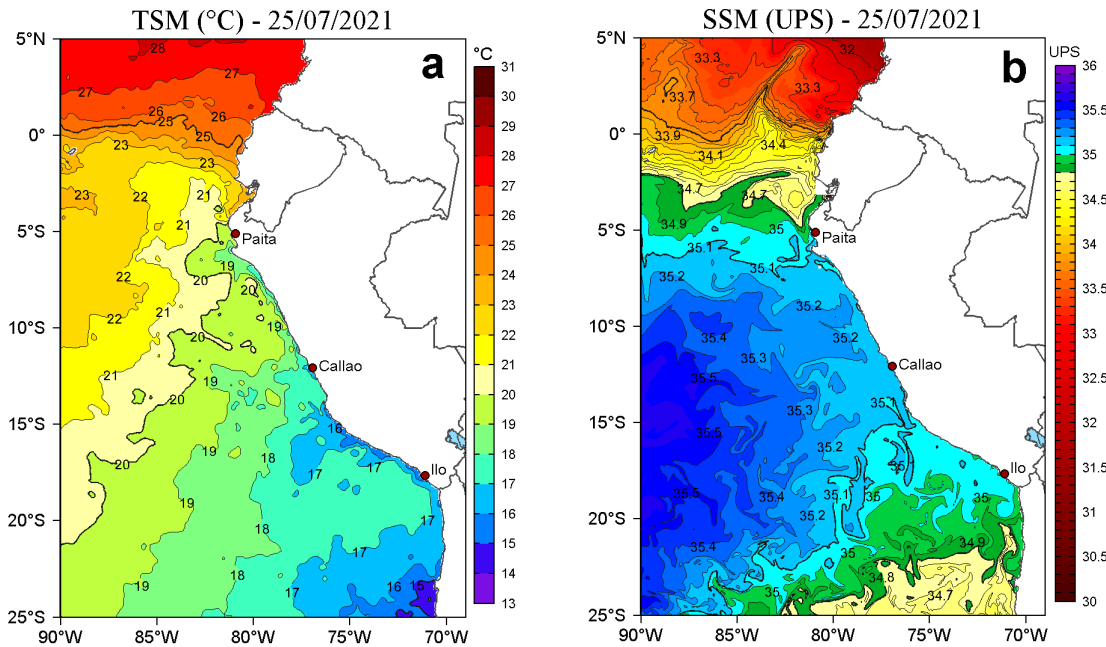
Figura 2. a) Temperatura superficial del mar (TSM, °C) y b) Salinidad superficial del mar (SSM) para el 25 de julio de 2021. Datos: OSTIA-UKMO-L4-GLOB-v2.0 (UK Met Office, 2012; Donlon et al, 2012) disponible en https://podaac.jpl.nasa.gov/dataset/OSTIA-UKMO-L4-GLOB-v2.0 para (a) y Hybrid Coordinate Ocean Model v. GOF5 3.1 (HYCOM; Halliwell et al., 1998; 2000; Bleck, 2001) para (b).
