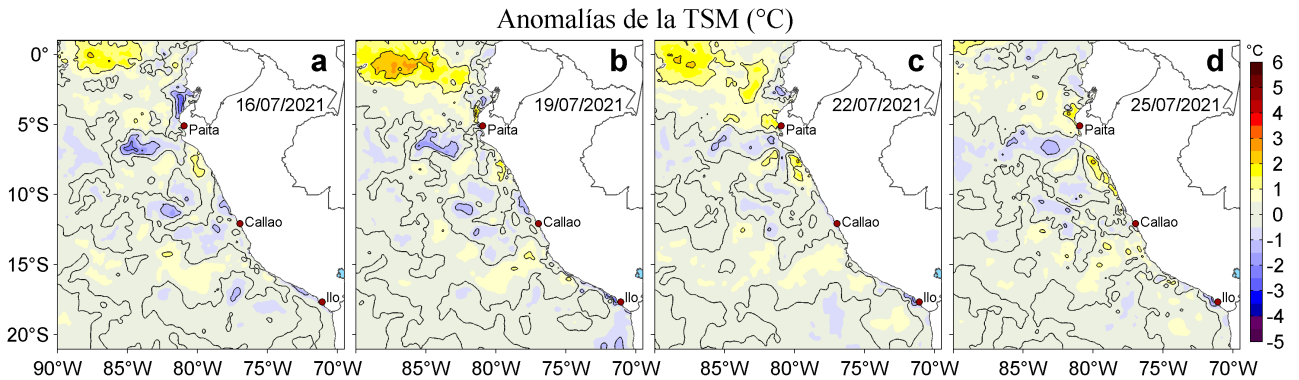
Figura 3. Anomalías de la temperatura superficial del mar (TSM, °C) para los días: a) 16, b) 19, c) 22 y d) 25 de julio de 2021. Las anomalías se calcularon respecto de la climatología para el periodo 2007-2016. Datos: OSTIA-UKMO-L4-GLOB-v2.0 (UK Met Office, 2012; Donlon et al, 2012).
