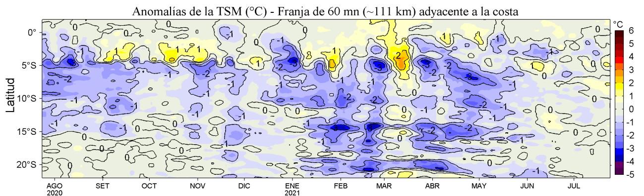
Figura 4. Variación promedio de las anomalías de la temperatura superficial del mar (TSM, °C) para una franja de 60 m.n. (~111 km) adyacente al litoral peruano para los últimos doce meses al 24 de julio de 2021. Datos: OSTIA-UKMO-L4-GLOB-v2.0 (UK Met. Office, 2012; Donlon et al, 2012) disponible en https://podaac.jpl.nasa.gov/dataset/OSTIA-UKMO-L4-GLOB-v2.0 . Las anomalías se calcularon con respecto al periodo 2007-2016.
