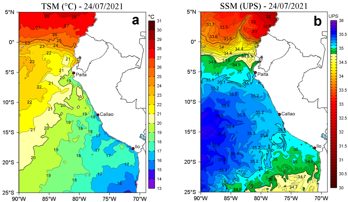
Figura 2. a) Temperatura superficial del mar (TSM, °C) y b) Salinidad superficial del mar (SSM) para el 24 de julio de 2021. Datos: OSTIA-UKMO-L4-GLOB-v2.0 (UK Met Office, 2012; Donlon et al, 2012) disponible en https://podaac.jpl.nasa.gov/dataset/OSTIA-UKMO-L4-GLOB-v2.0 para (a) y Hybrid Coordinate Ocean Model v. GOF5 3.1 (HYCOM; Halliwell et al., 1998; 2000; Bleck, 2001) para (b).
