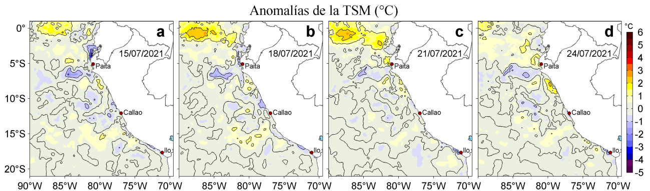
Figura 3. Anomalías de la temperatura superficial del mar (TSM, °C) para los días: a) 15, b) 18, c) 21 y d) 24 de julio de 2021. Las anomalías se calcularon respecto de la climatología para el periodo 2007-2016. Datos: OSTIA-UKMO-L4-GLOB-v2.0 (UK Met Office, 2012; Donlon et al, 2012).
