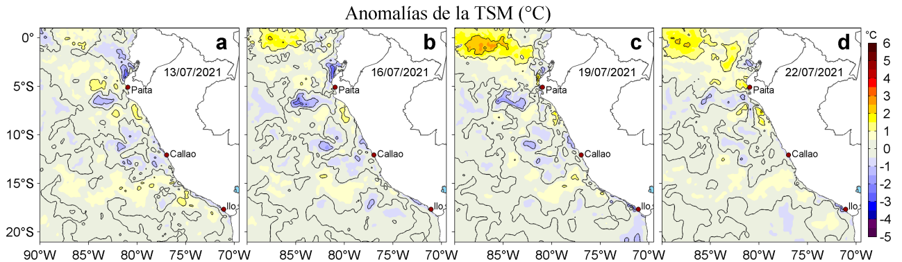
Figura 3. Anomalías de la temperatura superficial del mar (TSM, °C) para los días: a) 13, b) 16, c) 19 y d) 22 de julio de 2021. Las anomalías se calcularon respecto de la climatología para el periodo 2007-2016. Datos: OSTIA-UKMO-L4-GLOB-v2.0 (UK Met Office, 2012; Donlon et al, 2012).
