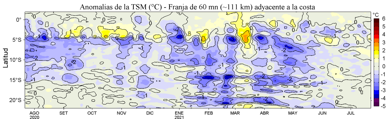
Figura 4. Variación promedio de las anomalías de la temperatura superficial del mar (TSM, °C) para una franja de 60 m.n. (~111 km) adyacente al litoral peruano para los últimos doce meses al 22 de julio de 2021. Datos: OSTIA-UKMO-L4-GLOB-v2.0 (UK Met. Office, 2012; Donlon et al, 2012) disponible en https://podaac.jpl.nasa.gov/dataset/OSTIA-UKMO-L4-GLOB-v2.0 . Las anomalías se calcularon con respecto al periodo 2007-2016.
