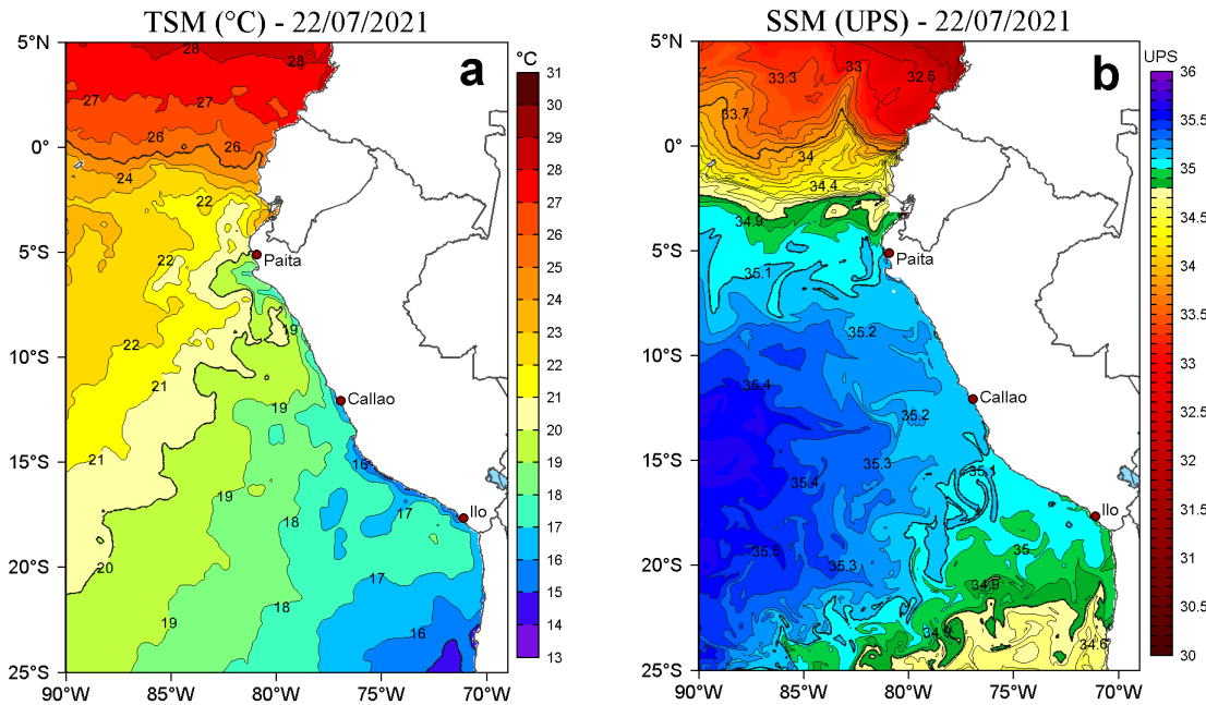
Figura 2. a) Temperatura superficial del mar (TSM, °C) y b) Salinidad superficial del mar (SSM) para el 22 de julio de 2021. Datos: OSTIA-UKMO-L4-GLOB-v2.0 (UK Met Office, 2012; Donlon et al, 2012) disponible en https://podaac.jpl.nasa.gov/dataset/OSTIA-UKMO-L4-GLOB-v2.0 para (a) y Hybrid Coordinate Ocean Model v. GOF3.1 (HYCOM; Halliwell et al., 1998; 2000; Bleck, 2001) para (b).
