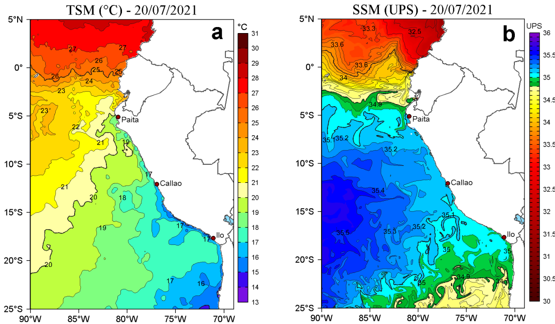
Figura 2. a) Temperatura superficial del mar (TSM, °C) y b) Salinidad superficial del mar (SSM) para el 20 de julio de 2021. Datos: OSTIA-UKMO-L4-GLOB-v2.0 (UK Met Office, 2012; Donlon et al, 2012) disponible en https://podaac.jpl.nasa.gov/dataset/OSTIA-UKMO-L4-GLOB-v2.0 para (a) y Hybrid Coordinate Ocean Model v. GOF5 3.1 (HYCOM; Halliwell et al., 1998; 2000; Bleck, 2001) para (b).
