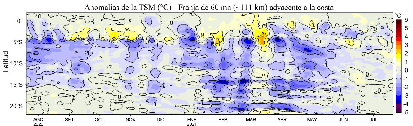
Figura 4. Variación promedio de las anomalías de la temperatura superficial del mar (TSM, °C) para una franja de 60 m.n. (~111 km) adyacente al litoral peruano para los últimos doce meses al 20 de julio de 2021. Datos: OSTIA-UKMO-L4-GLOB-v2.0 (UK Met. Office, 2012; Donlon et al, 2012) disponible en https://podaac.jpl.nasa.gov/dataset/OSTIA-UKMO-L4-GLOB-v2.0 . Las anomalías se calcularon con respecto al periodo 2007-2016.
