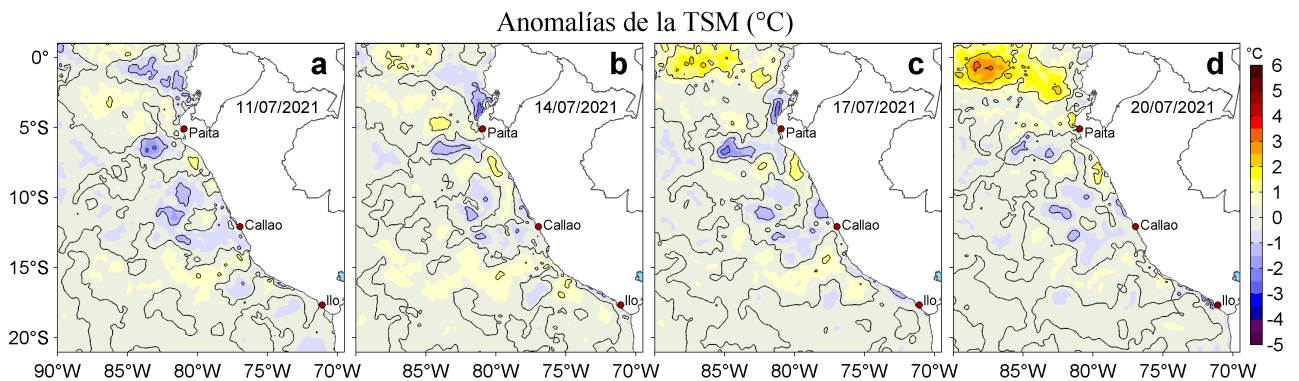
Figura 3. Anomalías de la temperatura superficial del mar (TSM, °C) para los días: a) 11, b) 14, c) 17 y d) 20 de julio de 2021. Las anomalías se calcularon respecto de la climatología para el periodo 2007-2016. Datos: OSTIA-UKMO-L4-GLOB-v2.0 (UK Met Office, 2012; Donlon et al, 2012).
