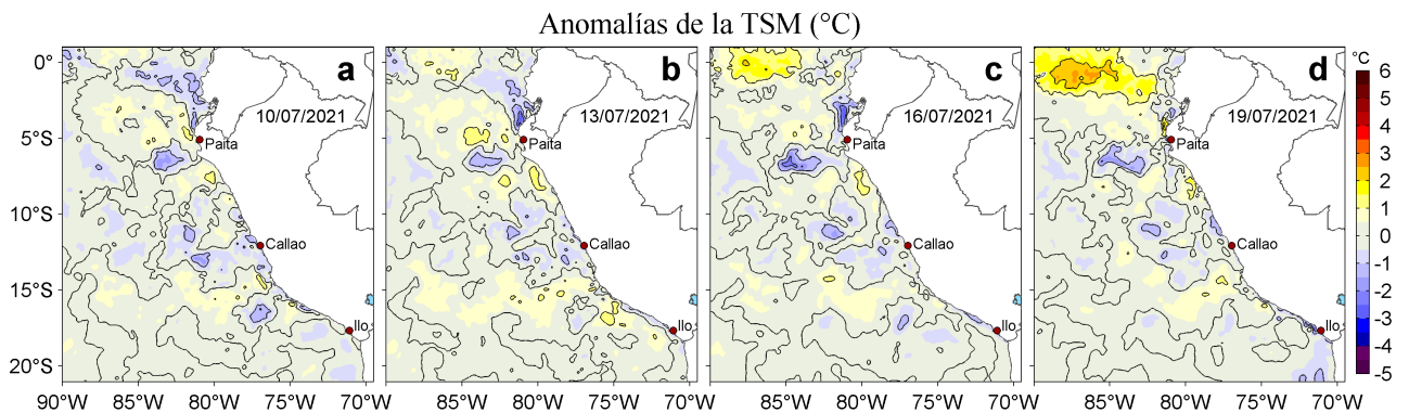
Figura 3. Anomalías de la temperatura superficial del mar (TSM, °C) para los días: a) 10, b) 13, c) 16 y d) 19 de julio de 2021. Las anomalías se calcularon respecto de la climatología para el periodo 2007-2016. Datos: OSTIA-UKMO-L4-GLOB-v2.0 (UK Met Office, 2012; Donlon et al, 2012).
