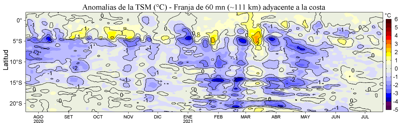
Figura 4. Variación promedio de las anomalías de la temperatura superficial del mar (TSM, °C) para una franja de 60 m.n. (~111 km) adyacente al litoral peruano para los últimos doce meses al 19 de julio de 2021. Datos: OSTIA-UKMO-L4-GLOB-v2.0 (UK Met. Office, 2012; Donlon et al, 2012) disponible en https://podaac.jpl.nasa.gov/dataset/OSTIA-UKMO-L4-GLOB-v2.0 . Las anomalías se calcularon con respecto al periodo 2007-2016.
