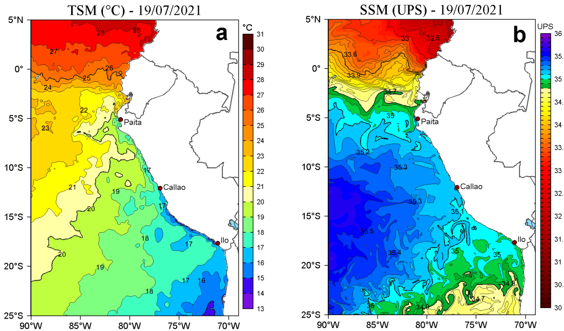
Figura 2. a) Temperatura superficial del mar (TSM, °C) y b) Salinidad superficial del mar (SSM) para el 19 de julio de 2021. Datos: OSTIA-UKMO-L4-GLOB-v2.0 (UK Met Office, 2012; Donlon et al, 2012) disponible en https://podaac.jpl.nasa.gov/dataset/OSTIA-UKMO-L4-GLOB-v2.0 para (a) y Hybrid Coordinate Ocean Model v. GOF5 3.1 (HYCOM; Halliwell et al., 1998; 2000; Bleck, 2001) para (b).
