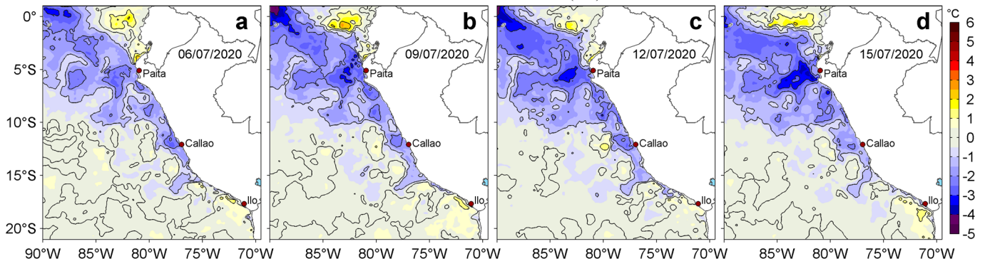
Figura 3. Anomalías de la temperatura superficial del mar (TSM, °C) para los días: a) 06, b) 09, c) 12 y d) 15 de julio de 2020. Las anomalías se calcularon respecto de la climatología para el periodo 2007-2016. Datos: OSTIA-UKMO-L4-GLOB-v2.0 (UK Met Office, 2012; Donlon et al, 2012). Procesamiento: LHF/AFIOF/DGIOCC/IMARPE.
