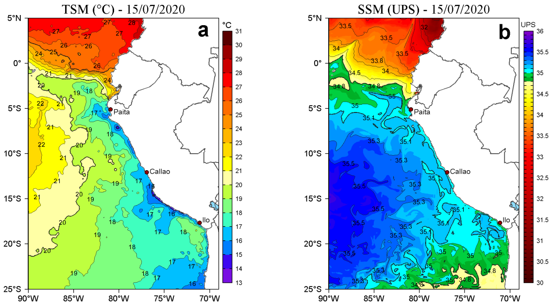
Figura 2. a) Temperatura superficial del mar (TSM, °C) y b) Salinidad superficial del mar (SSM, UPS), para el 15 de julio de 2020. Datos: OSTIA-UKMO-L4-GLOB-v2.0 (UK Met Office, 2012; Donlon et al, 2012) disponible en https://podaac.jpl.nasa.gov/dataset/OSTIA-UKMO-L4-GLOB-v2.0 para (a) y Hybrid Coordinate Ocean Model v. GOFS 3.1 (HYCOM; Halliwell et al., 1998; 2000; Bleck, 2001) para (b). Procesamiento: LHF/AFIOF/DGIOCC/IMARPE.
