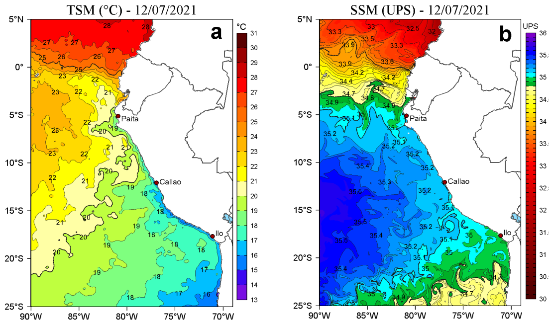
Figura 2. a) Temperatura superficial del mar (TSM, °C) y b) Salinidad superficial del mar (SSM) para el 12 de julio de 2021. Datos: OSTIA-UKMO-L4-GLOB-v2.0 (UK Met Office, 2012; Donlon et al, 2012) disponible en https://podaac.jpl.nasa.gov/dataset/OSTIA-UKMO-L4-GLOB-v2.0 para (a) y Hybrid Coordinate Ocean Model v. GOF5 3.1 (HYCOM; Halliwell et al., 1998; 2000; Bleck, 2001) para (b).
