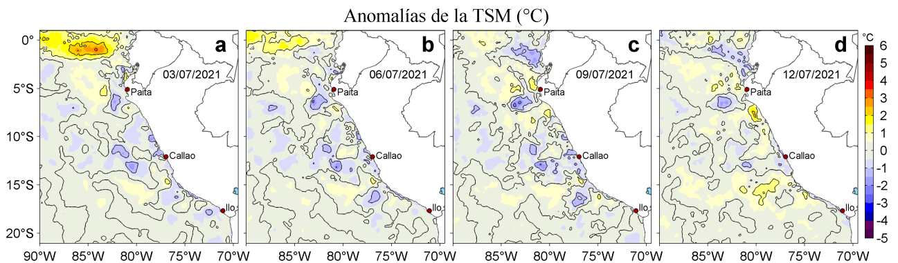
Figura 3. Anomalías de la temperatura superficial del mar (TSM, °C) para los días: a) 03, b) 06, c) 09 y d) 12 de julio de 2021. Las anomalías se calcularon respecto de la climatología para el periodo 2007-2016. Datos: OSTIA-UKMO-L4-GLOB-v2.0 (UK Met Office, 2012; Donlon et al, 2012).
