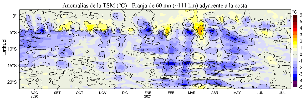
Figura 4. Variación promedio de las anomalías de la temperatura superficial del mar (TSM, °C) para una franja de 60 m.n. (~111 km) adyacente al litoral peruano para los últimos doce meses al 12 de julio de 2021. Datos: OSTIA-UKMO-L4-GLOB-v2.0 (UK Met. Office, 2012; Donlon et al, 2012) disponible en https://podaac.jpl.nasa.gov/dataset/OSTIA-UKMO-L4-GLOB-v2.0 . Las anomalías se calcularon con respecto al periodo 2007-2016.
