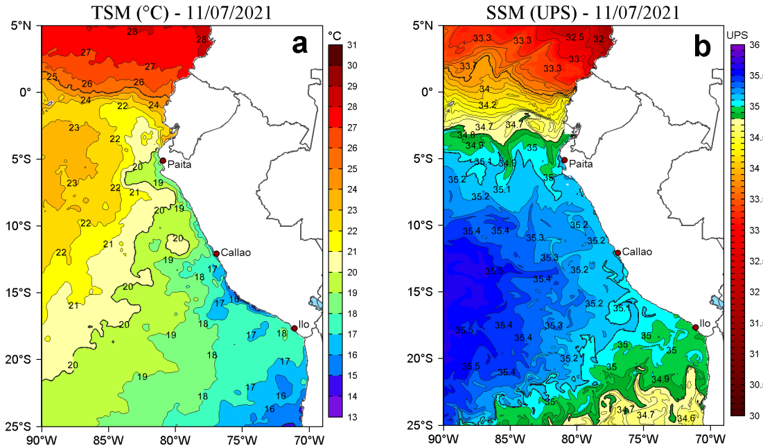
Figura 2. a) Temperatura superficial del mar (TSM, °C) y b) Salinidad superficial del mar (SSM) para el 11 de julio de 2021. Datos: OSTIA-UKMO-L4-GLOB-v2.0 (UK Met Office, 2012; Donlon et al, 2012) disponible en https://podaac.jpl.nasa.gov/dataset/OSTIA-UKMO-L4-GLOB-v2.0 para (a) y Hybrid Coordinate Ocean Model v. GOF5 3.1 (HYCOM; Halliwell et al., 1998; 2000; Bleck, 2001) para (b).
