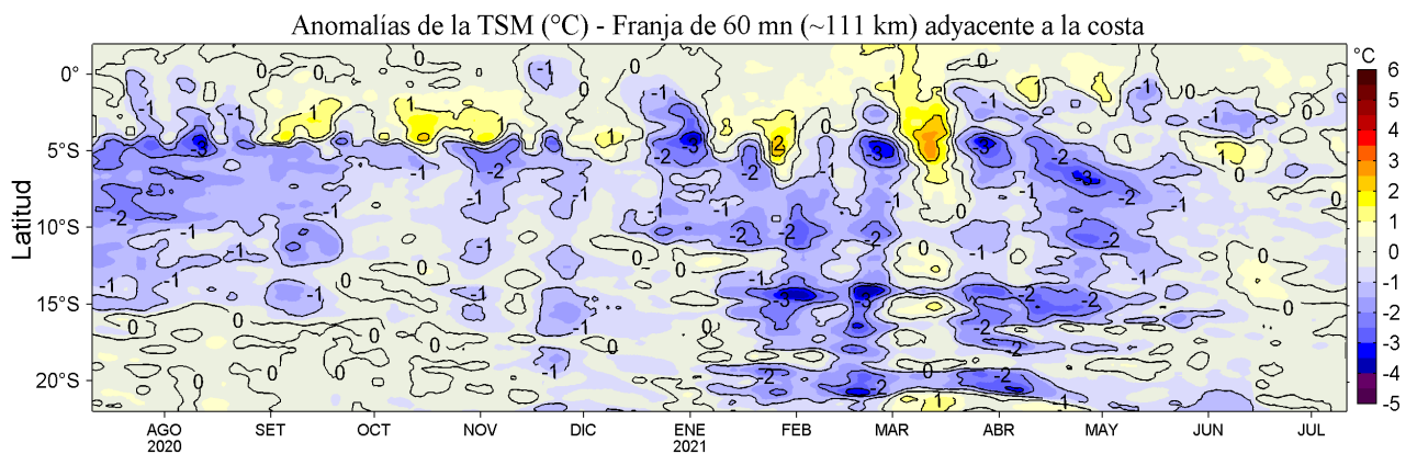
Figura 4. Variación promedio de las anomalías de la temperatura superficial del mar (TSM, °C) para una franja de 60 m.n. (~111 km) adyacente al litoral peruano para los últimos doce meses al 11 de julio de 2021. Datos: OSTIA-UKMO-L4-GLOB-v2.0 (UK Met. Office, 2012; Donlon et al, 2012) disponible en https://podaac.jpl.nasa.gov/dataset/OSTIA-UKMO-L4-GLOB-v2.0 . Las anomalías se calcularon con respecto al periodo 2007-2016.
