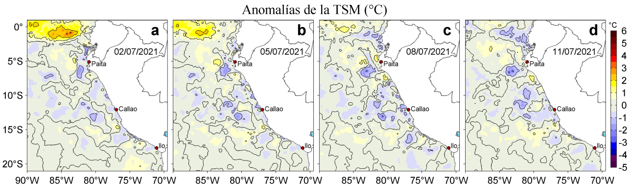
Figura 3. Anomalías de la temperatura superficial del mar (TSM, °C) para los días: a) 02, b) 05, c) 08 y d) 11 de julio de 2021. Las anomalías se calcularon respecto de la climatología para el periodo 2007-2016. Datos: OSTIA-UKMO-L4-GLOB-v2.0 (UK Met Office, 2012; Donlon et al, 2012).
