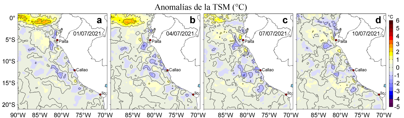
Figura 3. Anomalías de la temperatura superficial del mar (TSM, °C) para los días: a) 01, b) 04, c) 07 y d) 10 de julio de 2021. Las anomalías se calcularon respecto de la climatología para el periodo 2007-2016. Datos: OSTIA-UKMO-L4-GLOB-v2.0 (UK Met Office, 2012; Donlon et al, 2012).
