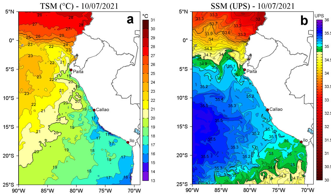
Figura 2. a) Temperatura superficial del mar (TSM, °C) y b) Salinidad superficial del mar (SSM) para el 10 de julio de 2021. Datos: OSTIA-UKMO-L4-GLOB-v2.0 (UK Met Office, 2012; Donlon et al, 2012) disponible en https://podaac.jpl.nasa.gov/dataset/OSTIA-UKMO-L4-GLOB-v2.0 para (a) y Hybrid Coordinate Ocean Model v. GOF5 3.1 (HYCOM; Halliwell et al., 1998; 2000; Bleck, 2001) para (b).
