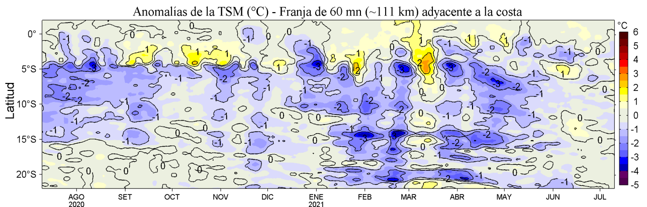
Figura 4. Variación promedio de las anomalías de la temperatura superficial del mar (TSM, °C) para una franja de 60 m.n. (~111 km) adyacente al litoral peruano para los últimos doce meses al 10 de julio de 2021. Datos: OSTIA-UKMO-L4-GLOB-v2.0 (UK Met. Office, 2012; Donlon et al, 2012) disponible en https://podaac.jpl.nasa.gov/dataset/OSTIA-UKMO-L4-GLOB-v2.0 . Las anomalías se calcularon con respecto al periodo 2007-2016.
