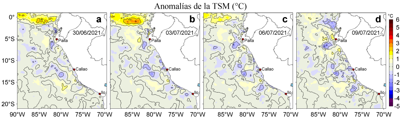
Figura 3. Anomalías de la temperatura superficial del mar (TSM, °C) para los días: a) 30 de junio, b) 03, c) 06 y d) 09 de julio de 2021. Las anomalías se calcularon respecto de la climatología para el periodo 2007-2016. Datos: OSTIA-UKMO-L4-GLOB-v2.0 (UK Met Office, 2012; Donlon et al, 2012).
