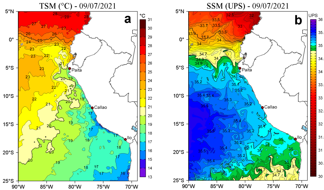
Figura 2. a) Temperatura superficial del mar (TSM, °C) y b) Salinidad superficial del mar (SSM) para el 09 de julio de 2021. Datos: OSTIA-UKMO-L4-GLOB-v2.0 (UK Met Office, 2012; Donlon et al, 2012) disponible en https://podaac.jpl.nasa.gov/dataset/OSTIA-UKMO-L4-GLOB-v2.0 para (a) y Hybrid Coordinate Ocean Model v. GOF5 3.1 (HYCOM; Halliwell et al., 1998; 2000; Bleck, 2001) para (b).
