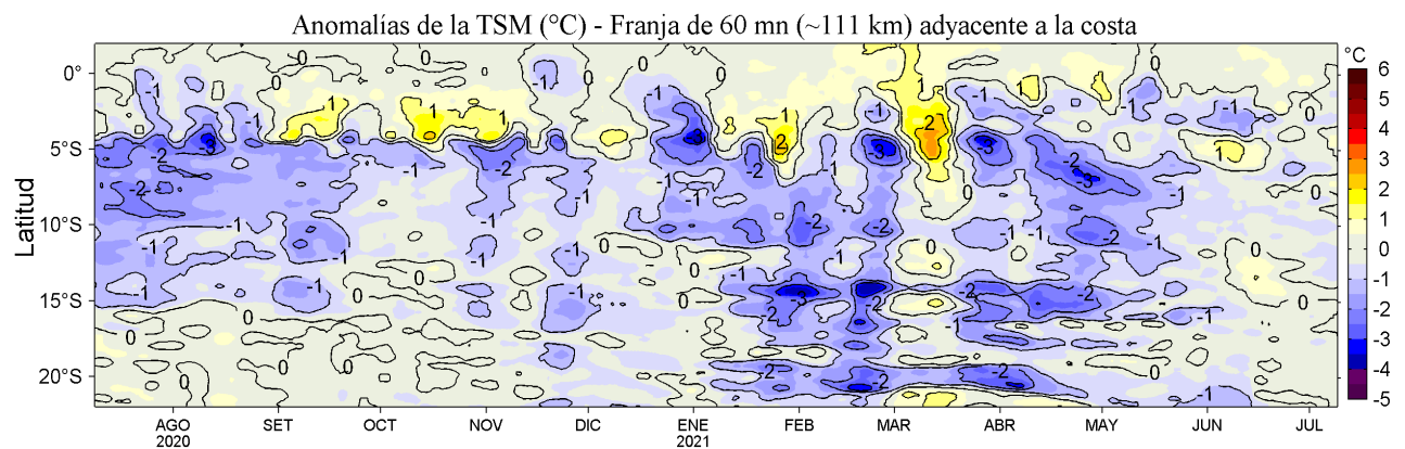
Figura 4. Variación promedio de las anomalías de la temperatura superficial del mar (TSM, °C) para una franja de 60 m.n. (~111 km) adyacente al litoral peruano para los últimos doce meses al 09 de julio de 2021. Datos: OSTIA-UKMO-L4-GLOB-v2.0 (UK Met. Office, 2012; Donlon et al, 2012) disponible en https://podaac.jpl.nasa.gov/dataset/OSTIA-UKMO-L4-GLOB-v2.0 . Las anomalías se calcularon con respecto al periodo 2007-2016.
