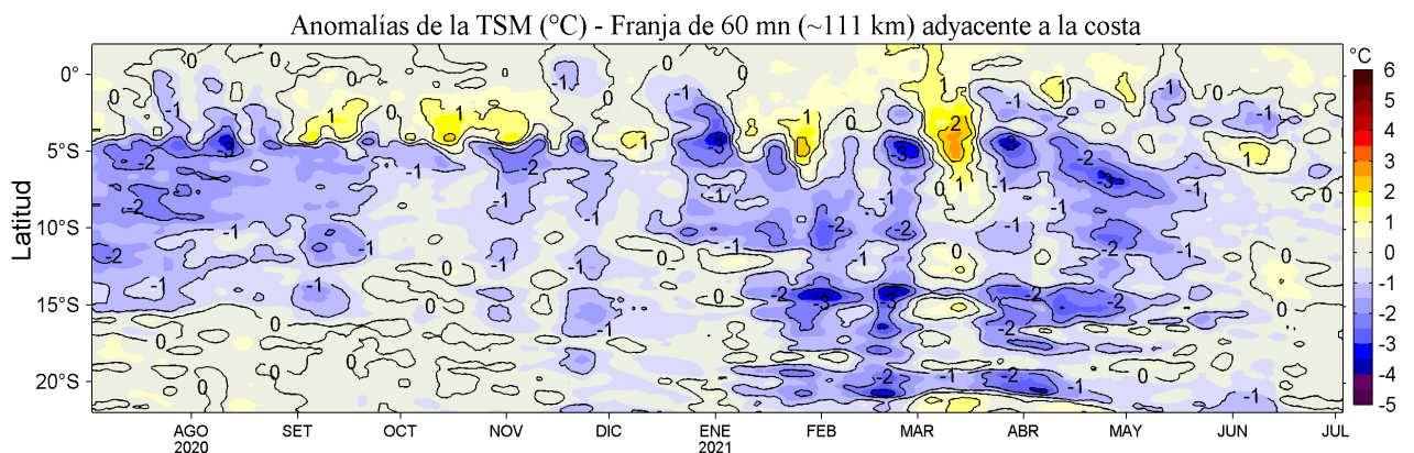
Figura 4. Variación promedio de las anomalías de la temperatura superficial del mar (TSM, °C) para una franja de 60 m.n. (~111 km) adyacente al litoral peruano para los últimos doce meses al 03 de julio de 2021. Datos: OSTIA-UKMO-L4-GLOB-v2.0 (UK Met. Office, 2012; Donlon et al, 2012) disponible en https://podaac.jpl.nasa.gov/dataset/OSTIA-UKMO-L4-GLOB-v2.0 . Las anomalías se calcularon con respecto al periodo 2007-2016.
