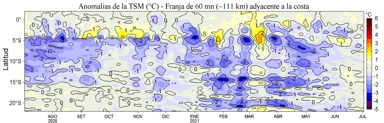
Figura 4. Variación promedio de las anomalías de la temperatura superficial del mar (TSM, °C) para una franja de 60 m.n. (~111 km) adyacente al litoral peruano para los últimos doce meses al 02 de julio de 2021. Datos: OSTIA-UKMO-L4-GLOB-v2.0 (UK Met. Office, 2012; Donlon et al, 2012) disponible en https://podaac.jpl.nasa.gov/dataset/OSTIA-UKMO-L4-GLOB-v2.0 . Las anomalías se calcularon con respecto al periodo 2007-2016.
