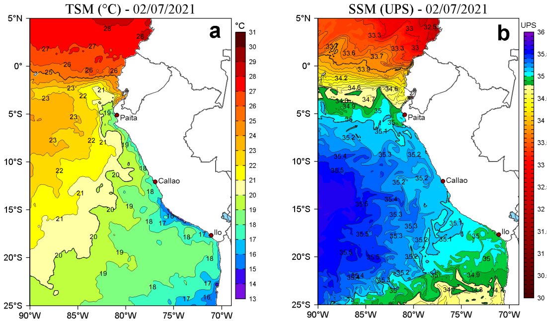
Figura 2. a) Temperatura superficial del mar (TSM, °C) y b) Salinidad superficial del mar (SSM) para el 02 de julio de 2021. Datos: OSTIA-UKMO-L4-GLOB-v2.0 (UK Met Office, 2012; Donlon et al, 2012) disponible en https://podaac.jpl.nasa.gov/dataset/OSTIA-UKMO-L4-GLOB-v2.0 para (a) y Hybrid Coordinate Ocean Model v. GOFS 3.1 (HYCOM; Halliwell et al., 1998; 2000; Bleck, 2001) para (b).
