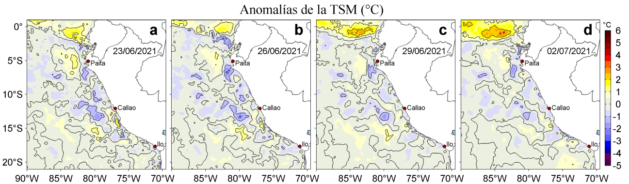
Figura 3. Anomalías de la temperatura superficial del mar (TSM, °C) para los días: a) 23, b) 26 y c) 29 de junio y d) 02 de julio de 2021. Las anomalías se calcularon respecto de la climatología para el periodo 2007-2016. Datos: OSTIA-UKMO-L4-GLOB-v2.0 (UK Met Office, 2012; Donlon et al, 2012).
